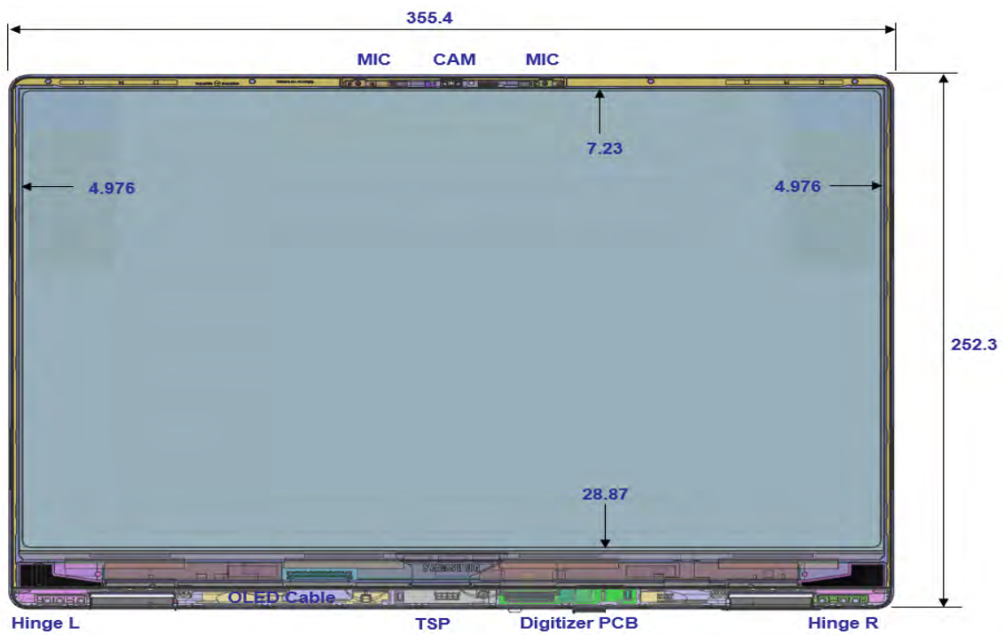
LCD_ASSY
