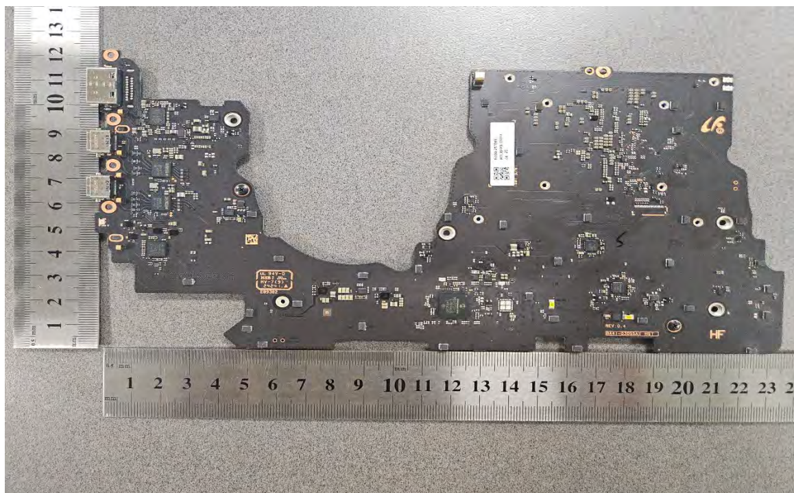
MBD Bottom
