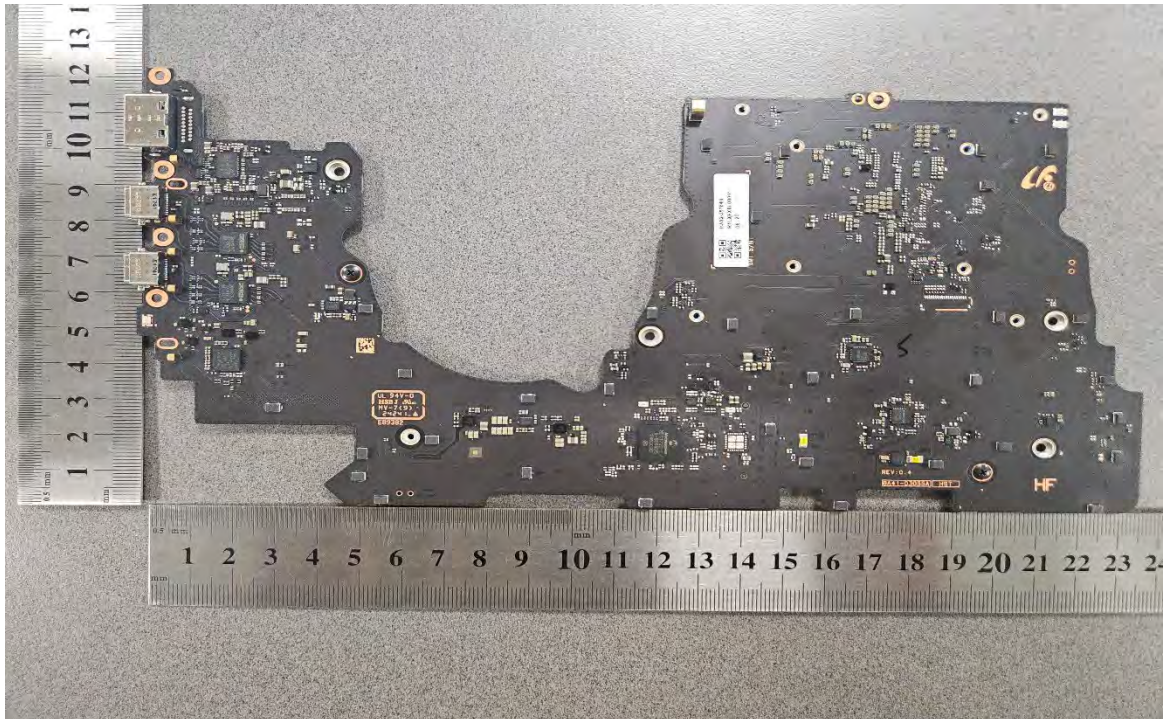
Inisde EUT#28
