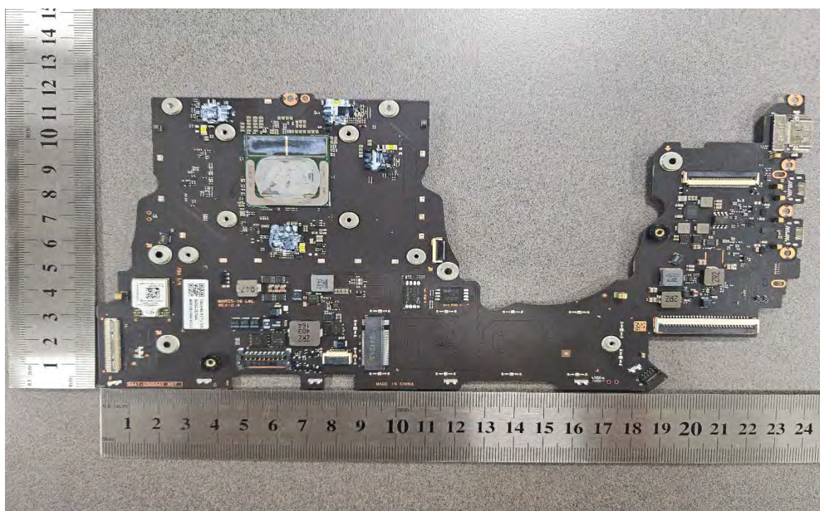
MBD Top
