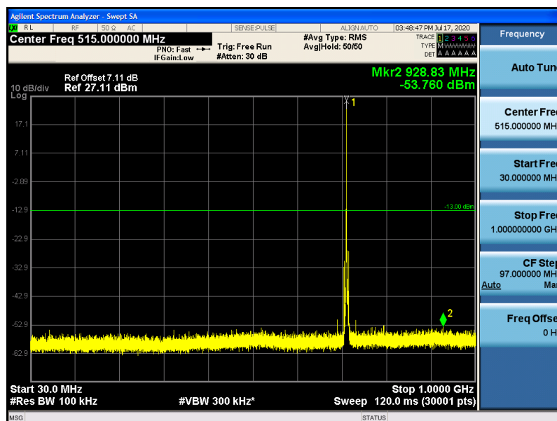
Band5-5MHz-QPSK-20425-1RB#0-30~1000MHz
