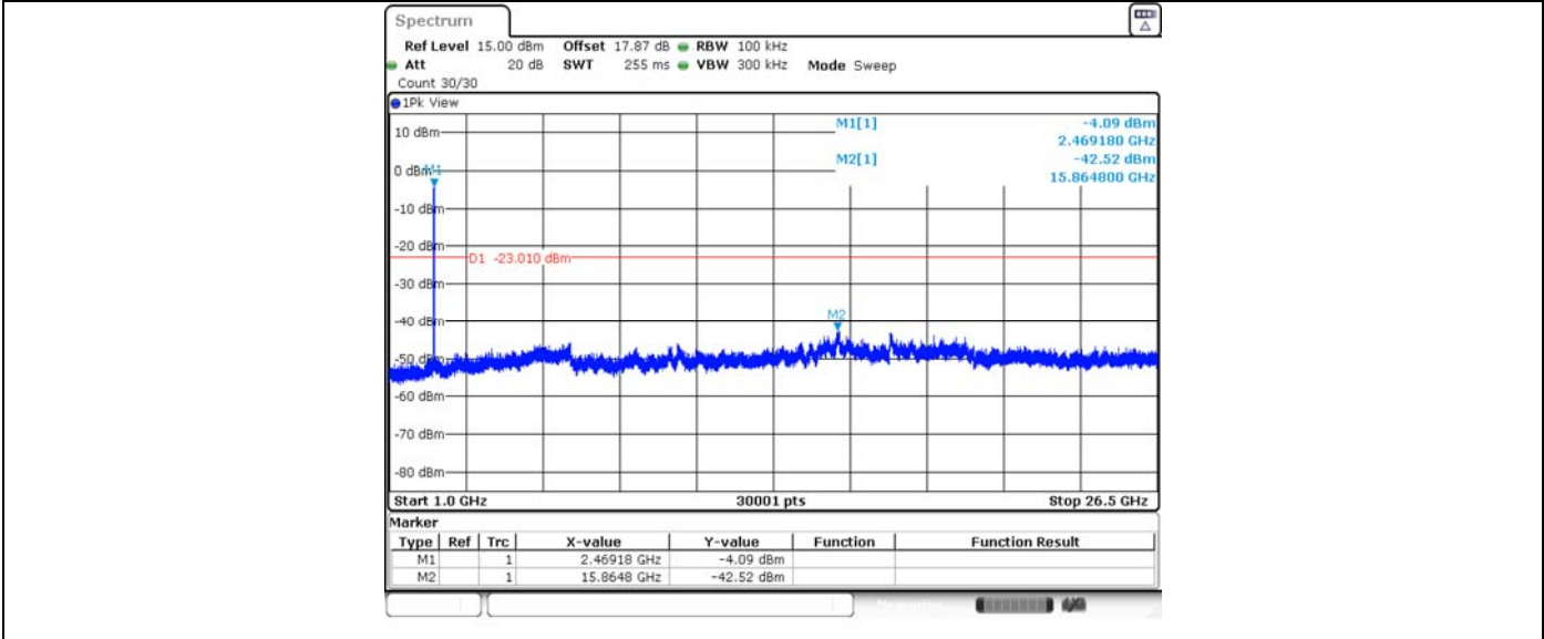
11N20MIMO_Ant2_2462_1000~26500
