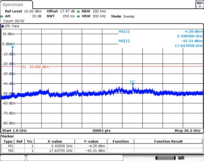
11N20MIMO_Ant2_2437_1000~26500
