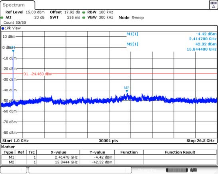
11N20MIMO_Ant1_2412_1000~26500
