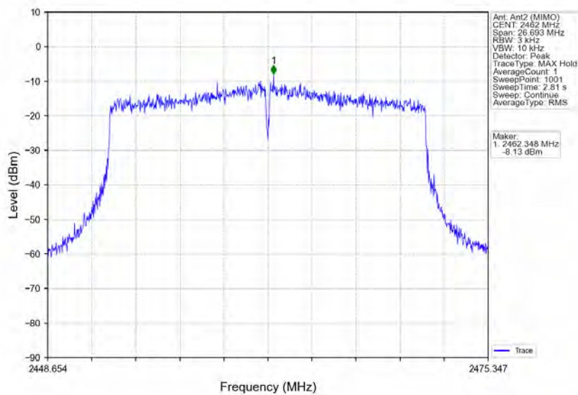
802.11ax(HEW20)_HCH_2462MHz_RU242_Left_Ant2 (MIMO)_NTNV
