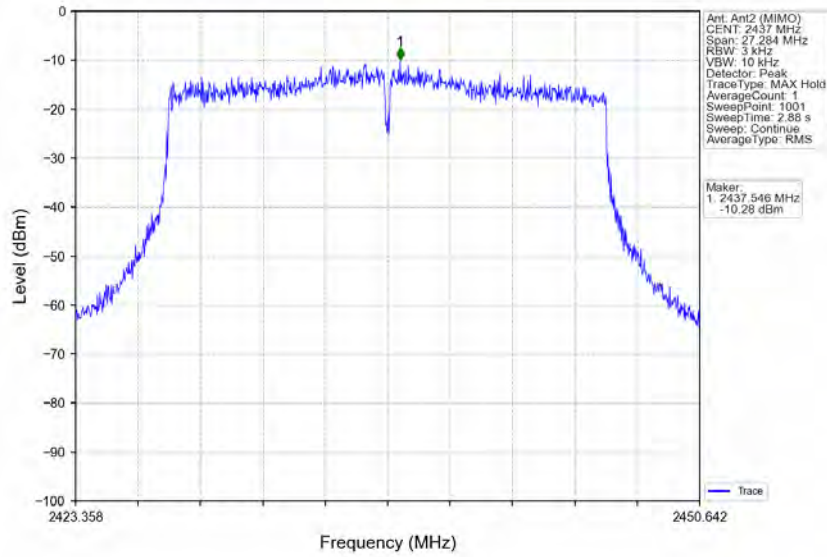
802.11ax(HEW20)_MCH_2437MHz_RU242_Left_MIMO_NTNV
