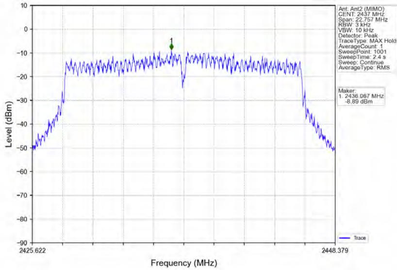
802.11n(HT20)_MCH_2437MHz_MIMO_NTNV
