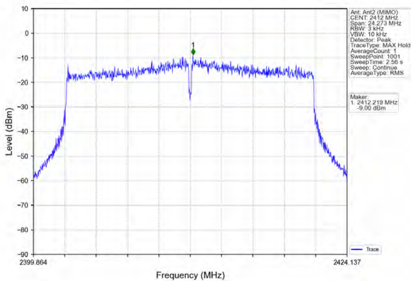
802.11ax(HEW20)_LCH_2412MHz_RU242_Left_Ant2 (MIMO)_NTNV
