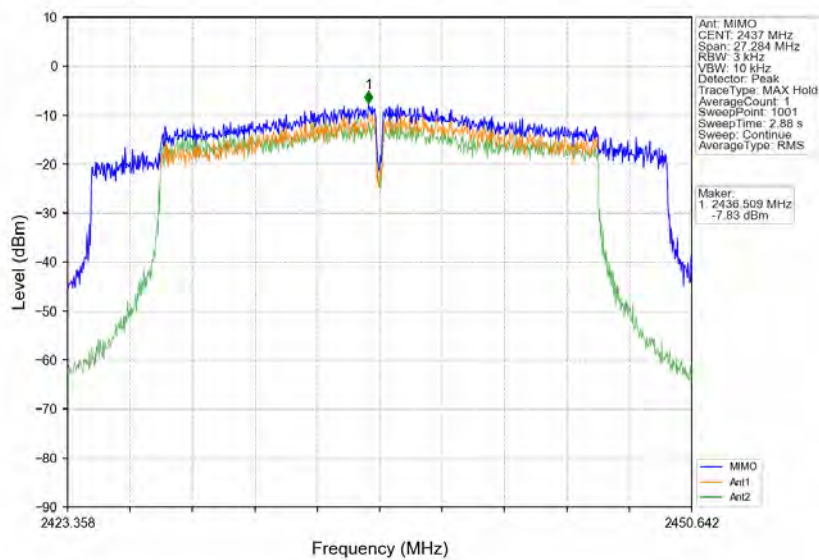
802.11ax(HEW20)_MCH_2437MHz_RU242_Left_MIMO_NTNV
