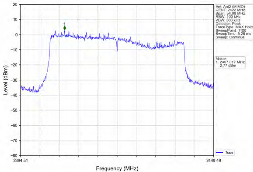
802.11ax(HEW40)_LCH_2422MHz_RU484_Left_Ant2 (MIMO)_NTNV
