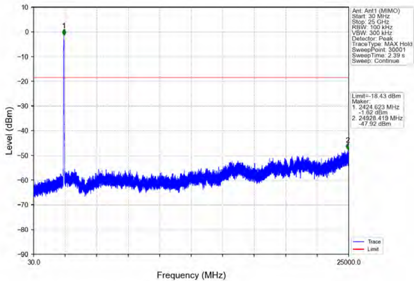
802.11ax(HEW40)_LCH_2422MHz_RU484_Left_Ant1 (MIMO)_NTNV
