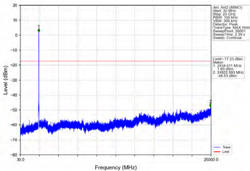
802.11ax(HEW40)_MCH_2437MHz_RU484_Left_Ant2 (MIMO)_NTNV
