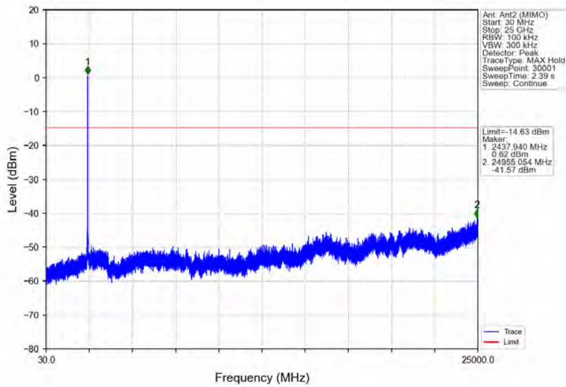
802.11ax(HEW20)_MCH_2437MHz_RU242_Left_Ant2 (MIMO)_NTNV
