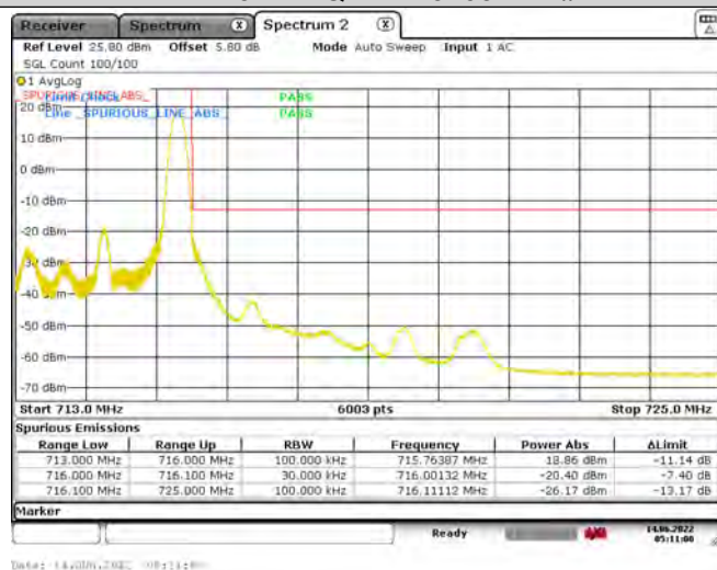
Band12-3MHz-QPSK-23165-15RB#0
