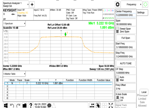
802.11ax_20MHz_Chain1_5220MHz
