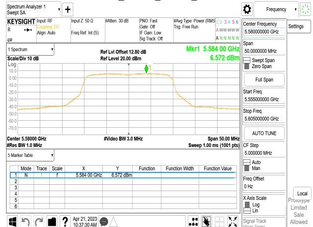
802.11ax_20MHz_Chain1_5580MHz
