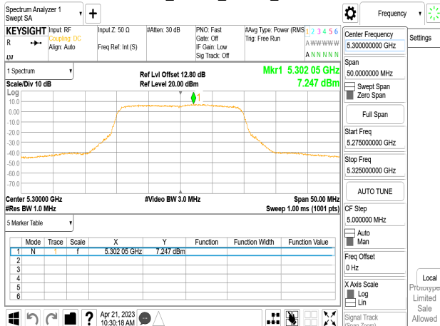
802.11ax_20MHz_Chain1_5300MHz
