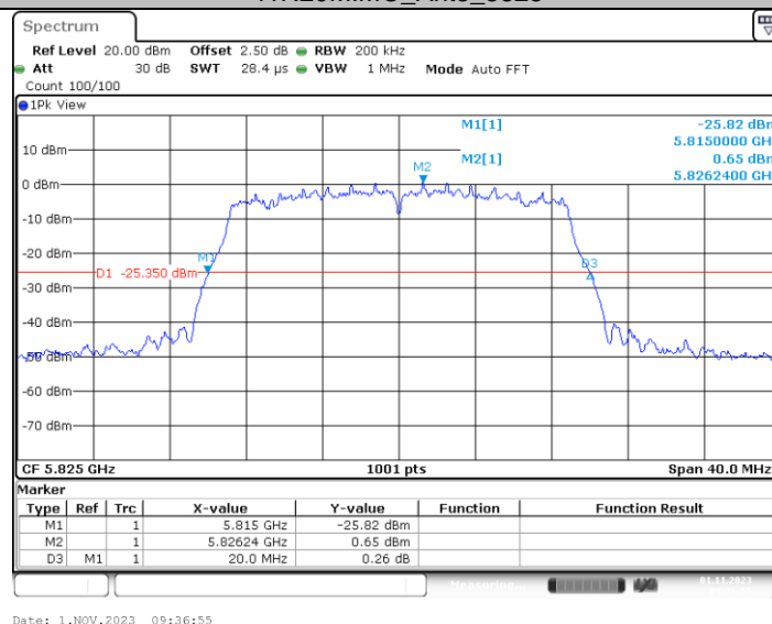
11N20MIMO_Ant4_5825
