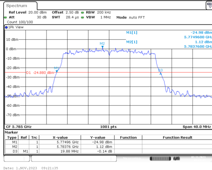
11N20MIMO_Ant3_5785
