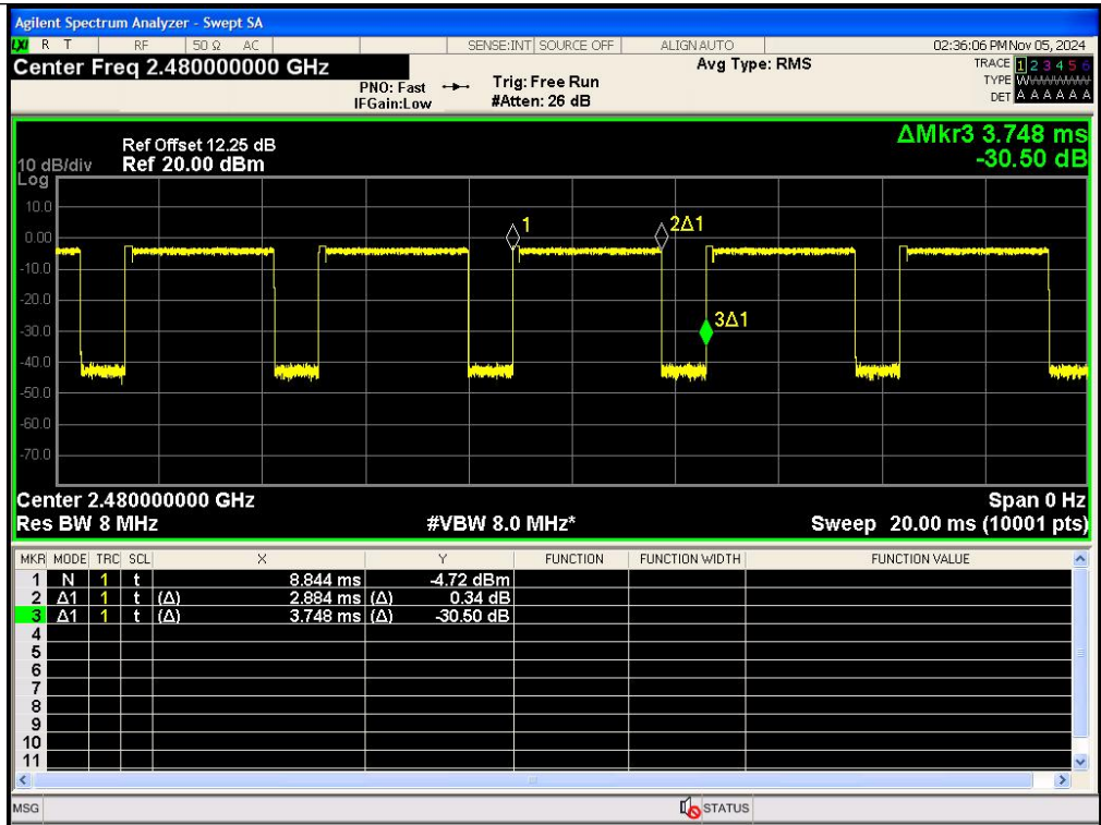
\pi/4 DQPSK(2-DH5)_Channel 78
