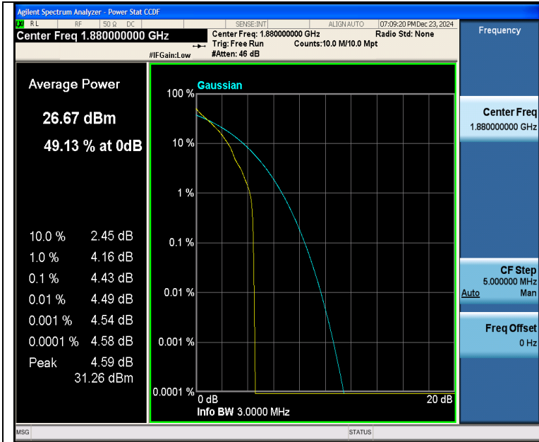
Band2-3MHz-QPSK-18900-1RB#0-PASS
