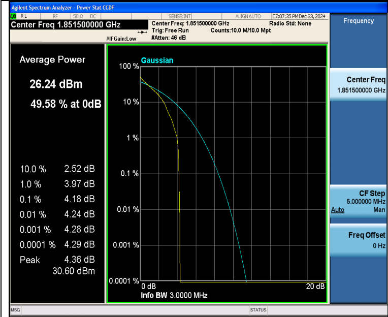
Band2-3MHz-QPSK-18615-1RB#0-PASS
