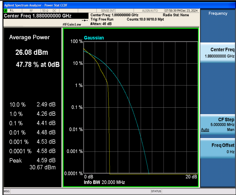
Band2-20MHz-QPSK-18900-1RB#0-PASS
