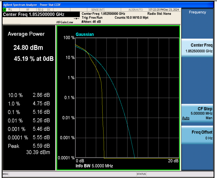
Band2-5MHz-16QAM-18625-1RB#0-PASS
