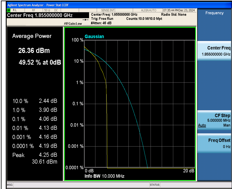
Band2-10MHz-QPSK-18650-1RB#0-PASS
