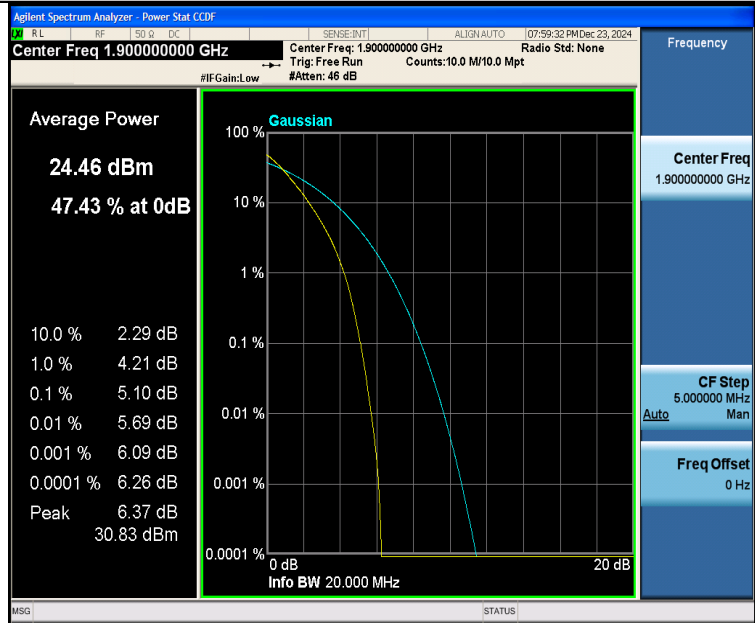
Band2-20MHz-QPSK-19100-100RB#0-PASS
