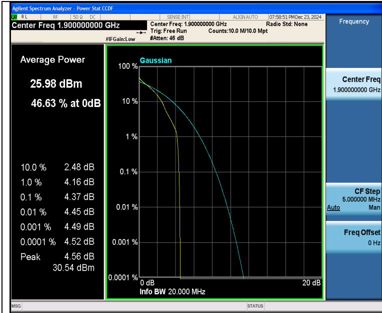
Band2-20MHz-QPSK-19100-1RB#0-PASS
