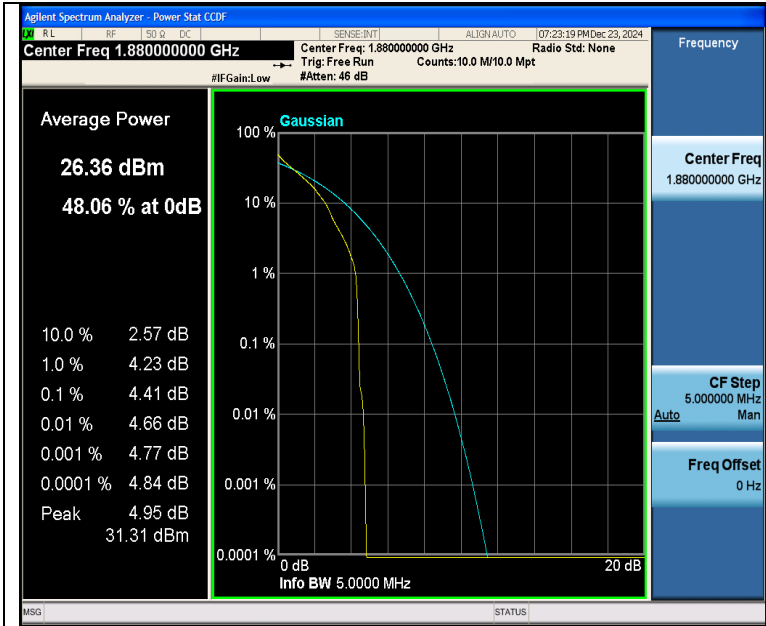
Band2-5MHz-QPSK-18900-1RB#0-PASS
