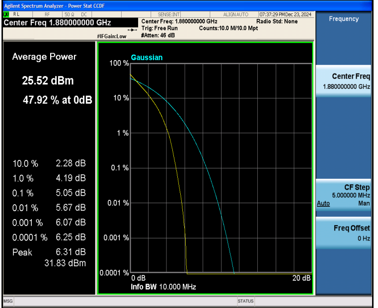
Band2-10MHz-QPSK-18900-50RB#0-PASS
