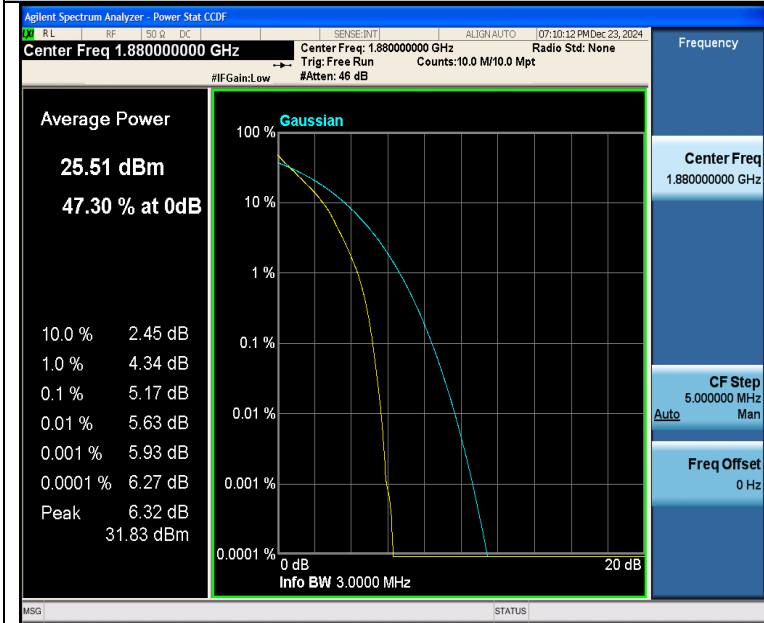
Band2-3MHz-QPSK-18900-15RB#0-PASS
