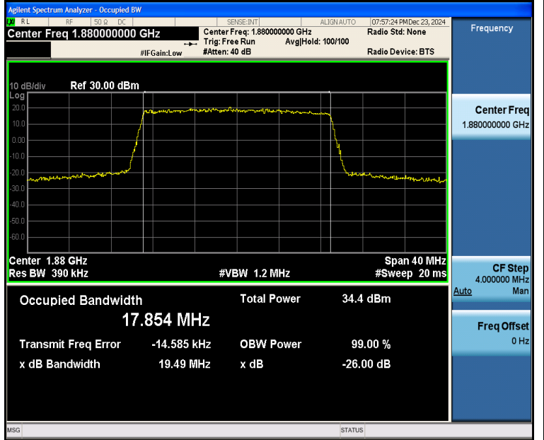
Band2-20MHz-QPSK-18900-100RB#0-PASS
