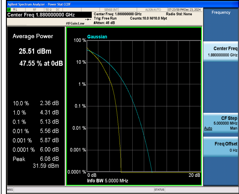
Band2-5MHz-QPSK-18900-25RB#0-PASS
