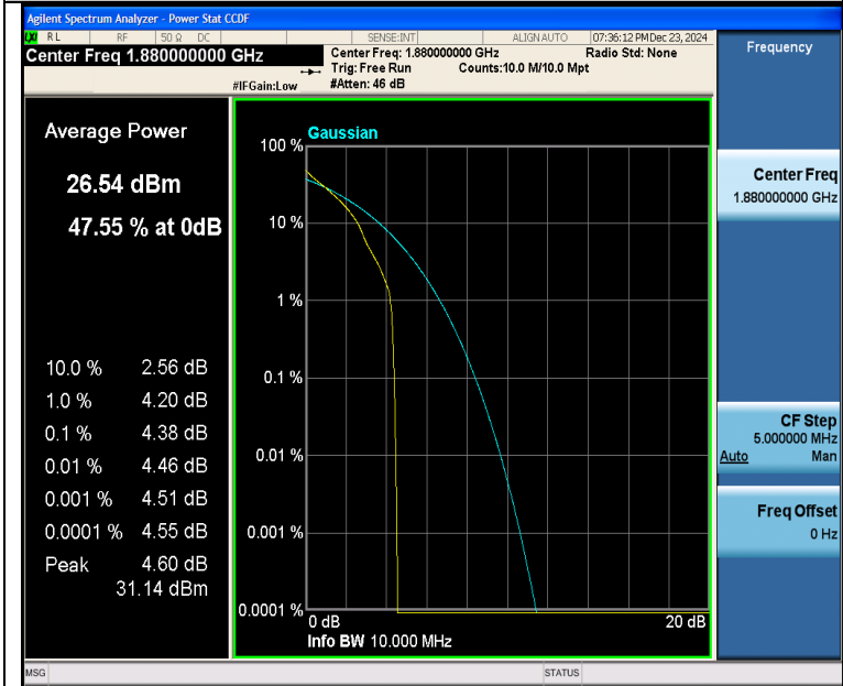
Band2-10MHz-QPSK-18900-1RB#0-PASS
