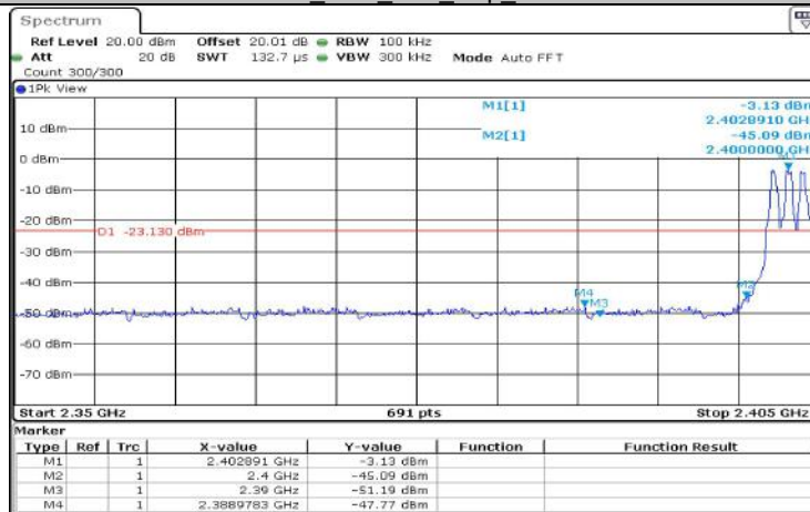
DH1_Ant1_Low_Hop_2402
