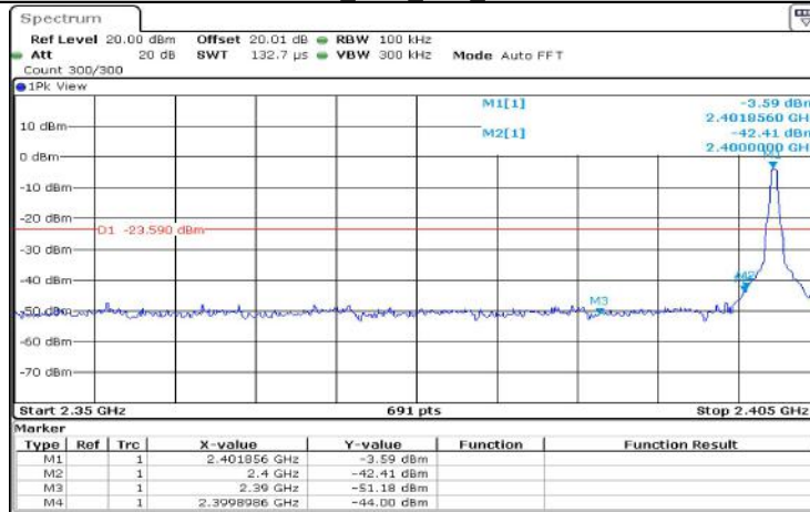
DH1_Ant1_Low_2402
