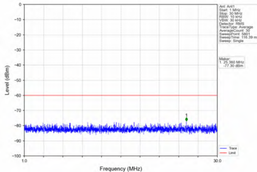
n78d_30kHz_SISO_NTNV_70MHz_CP-OFDM_QPSK_3585MHz_Inner_1RB_Left
