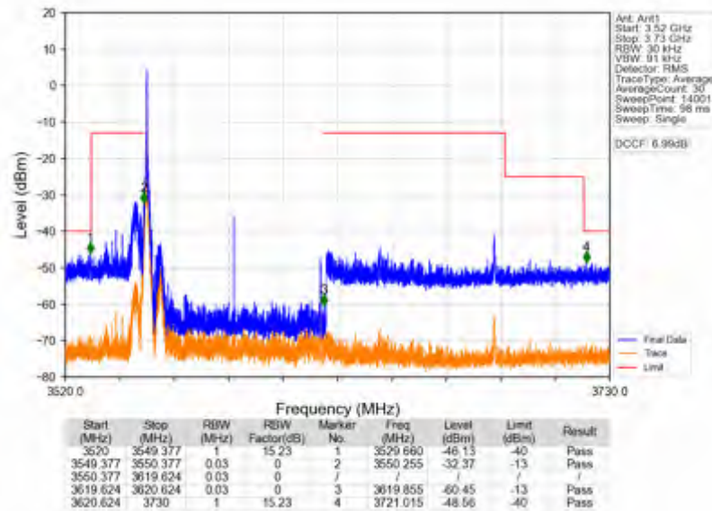
n78d_30kHz_SISO_NTV_70MHz_CP-OFDM_QPSK_3585MHz_Inner_1RB_Left
