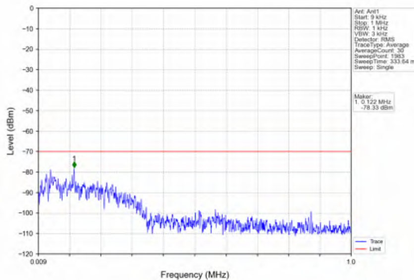
n78d_30kHz_SISO_NTV_70MHz_CP-OFDM_QPSK_3585MHz_Inner_1RB_Left
