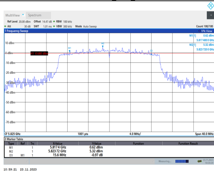
11AX20MIMO_Ant2_5825
