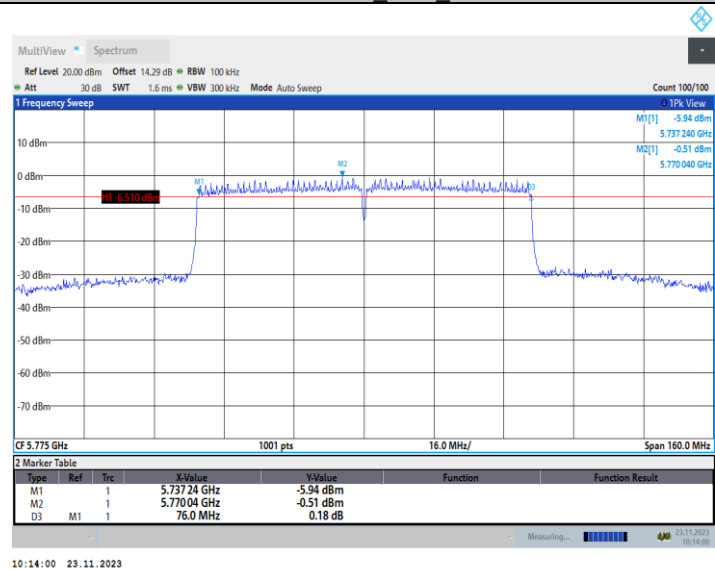
11AC80MIMO_Ant2_5775
