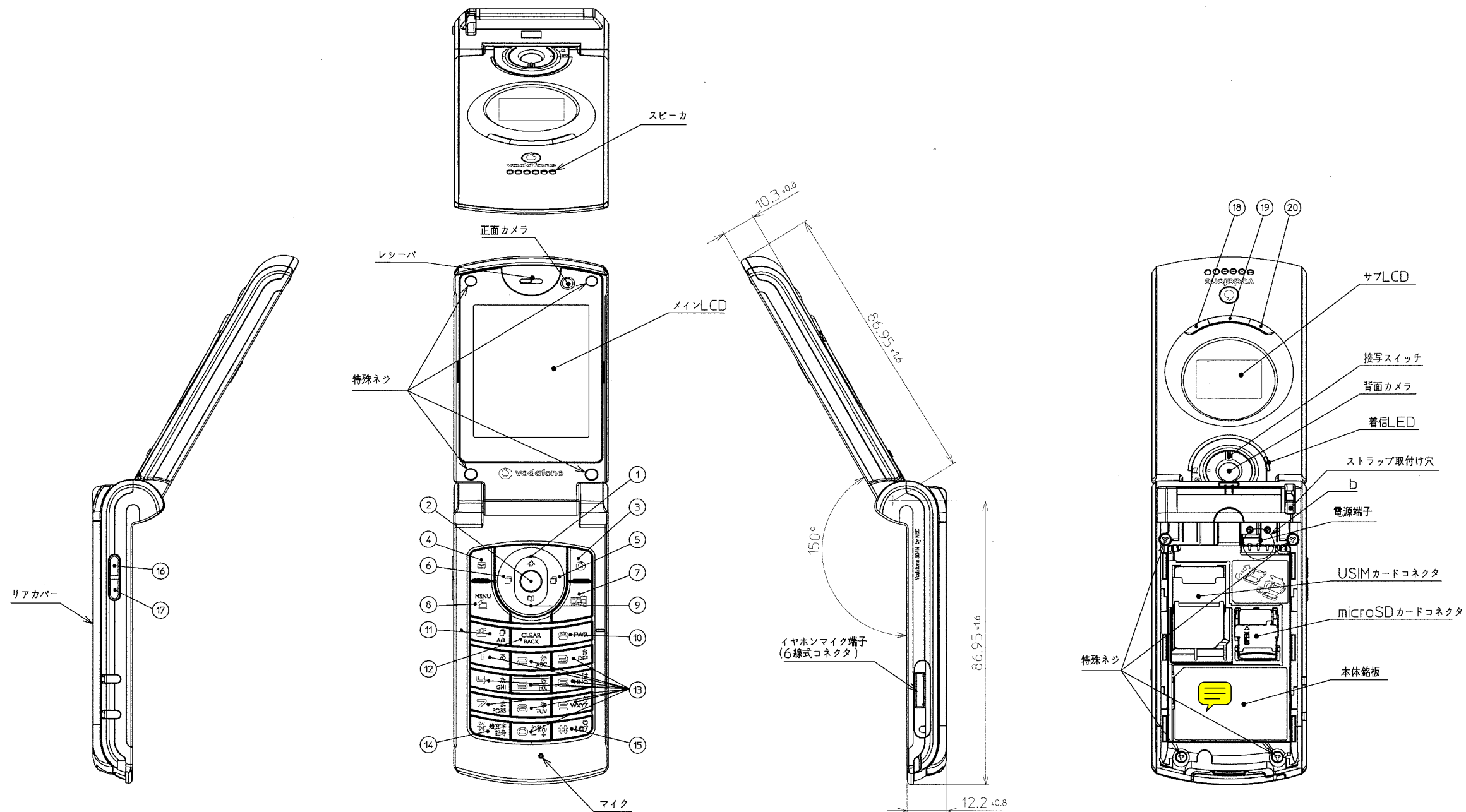
電池バック及びリアカバー装着時
