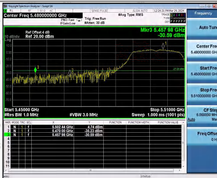
11AC20MIMO_Ant1_Low_5500
