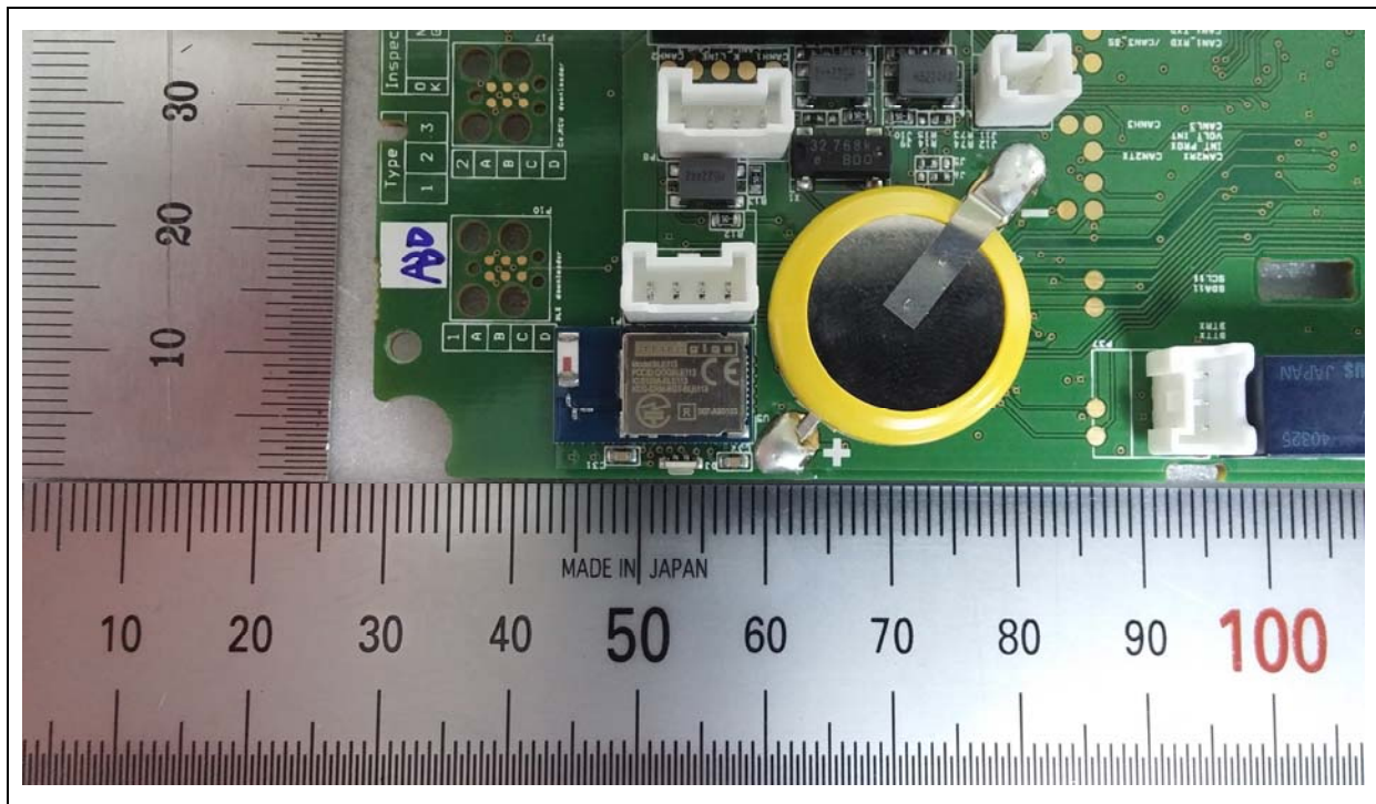
&lt;BT Antenna&gt;
