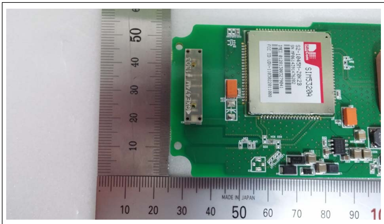
&lt;GSM Antenna&gt;
