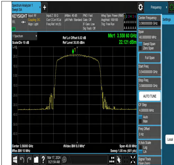
42(3550-3600)-20MHz-QPSK-43190-1RB#49-PASS
