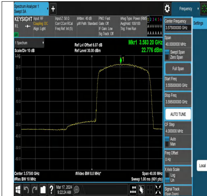
42(3550-3600)-20MHz-QPSK-43340-1RB#99-PASS
