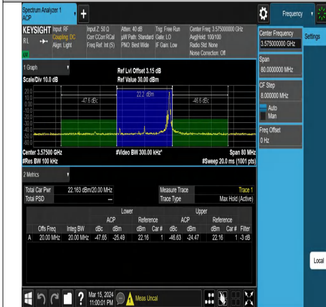
42(3550-3600)-20MHz-QPSK-43340-1RB#99-PASS
