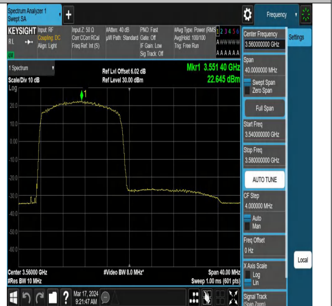
42(3550-3600)-20MHz-QPSK-43190-1RB#0-PASS
