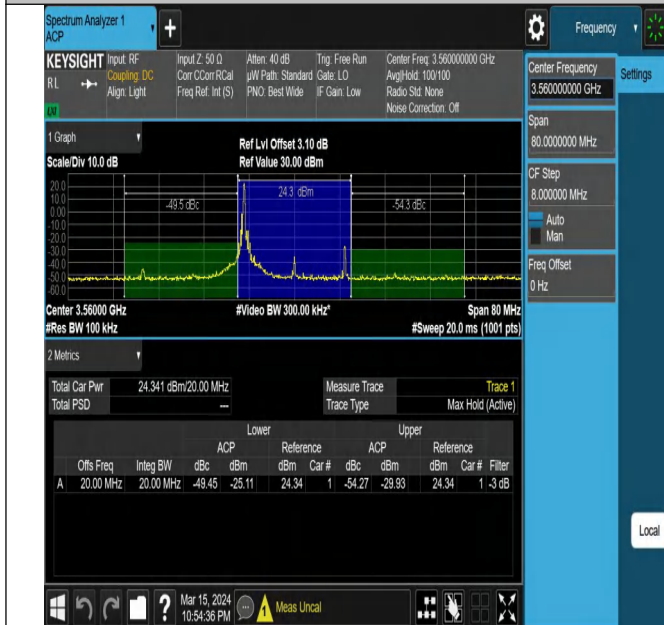
42(3550-3600)-20MHz-QPSK-43190-1RB#0-PASS
