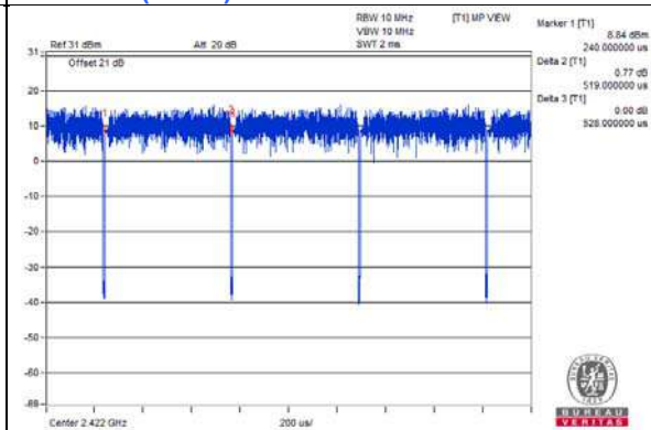
802.11ax (RU52)
