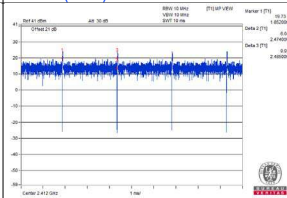
802.11ax (RU52)
