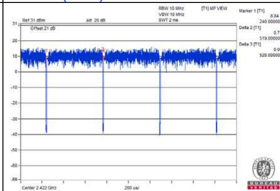
802.11ax (RU52)
