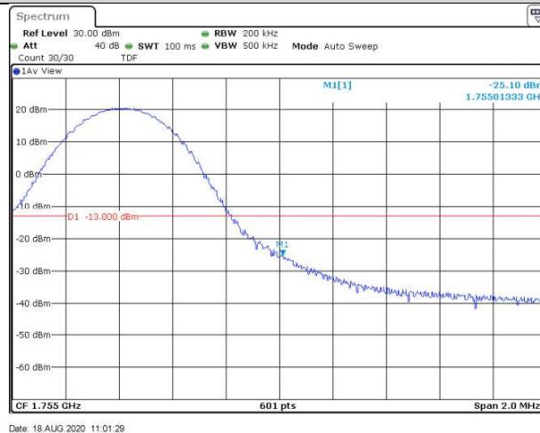
Band4-10MHz-QPSK-20350-1RB#0
