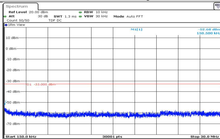
Band4-1.4MHz-QPSK-19957-1RB#0-Range2:0.15~30MHz
