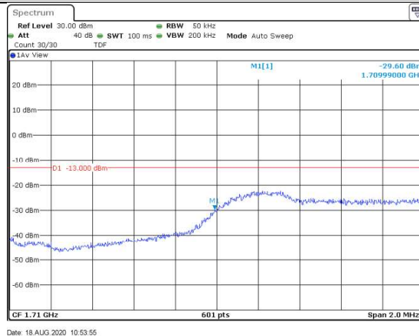
Band4-3MHz-QPSK-19965-1RB#0
