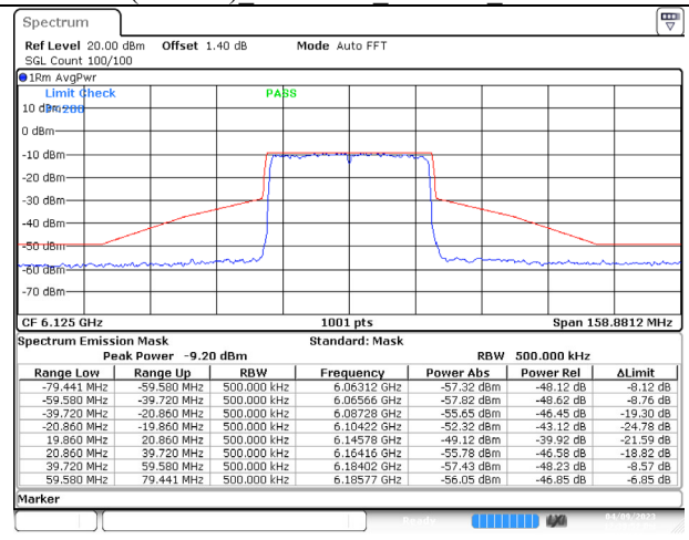
802.11ax (40MHz) 6125MHz Chain B NSS-4
