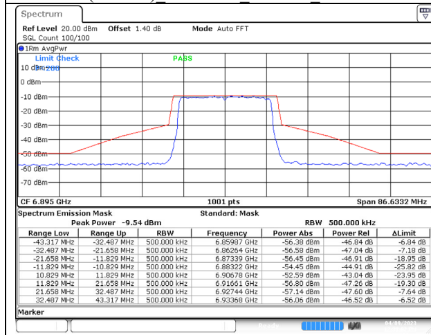
802.11ax (20MHz) 6895MHz Chain A NSS-4
