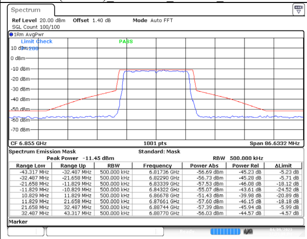
802.11ax (20MHz) 6855MHz Chain D NSS-4
