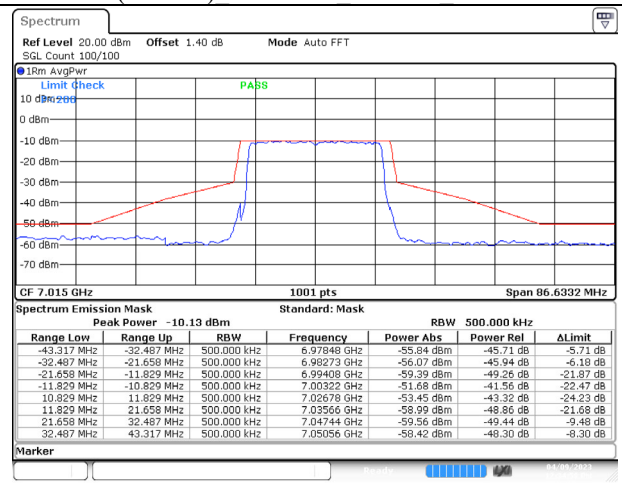
802.11ax (20MHz) 7015MHz Chain B NSS-4
