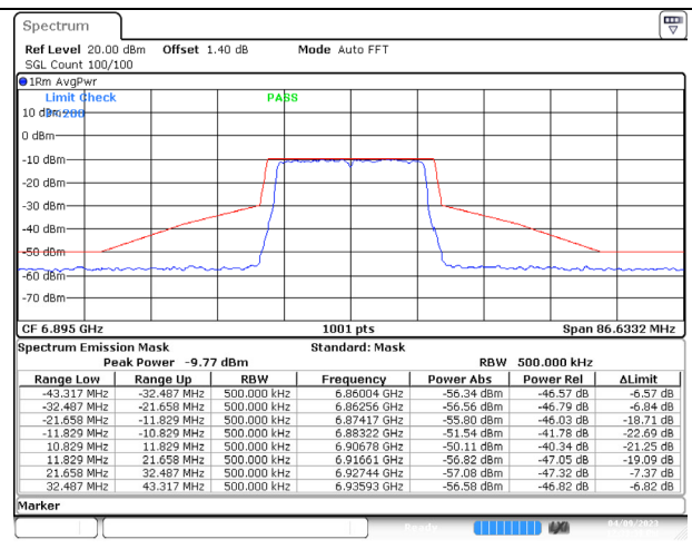
802.11ax (20MHz) 6895MHz Chain D NSS-4
