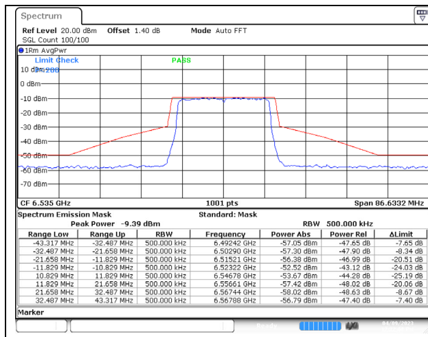
802.11ax (20MHz) 6535MHz Chain A NSS-4
