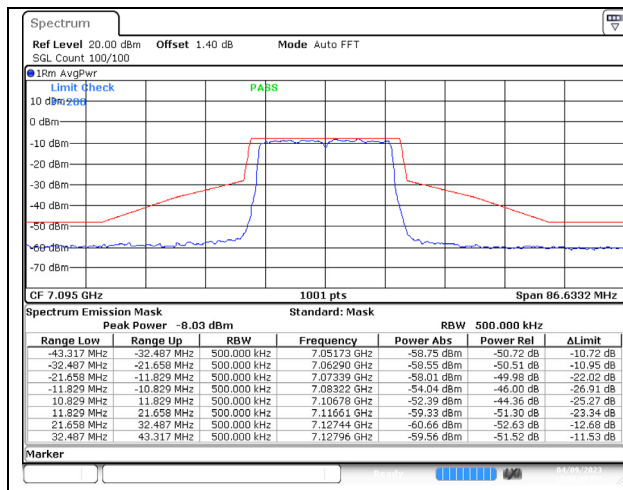
802.11ax (20MHz) 7095MHz Chain A NSS-4
