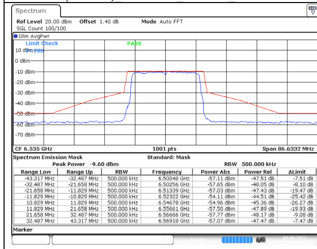
802.11ax (20MHz) 6535MHz Chain C NSS-4
