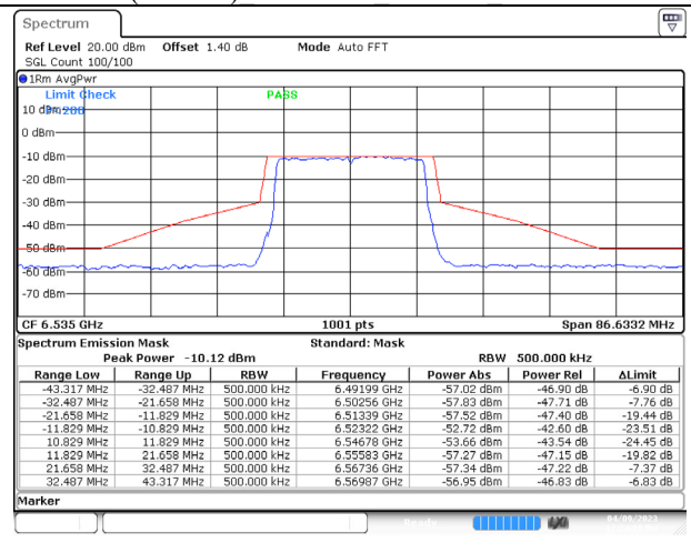
802.11ax (20MHz) 6535MHz Chain D NSS-4
