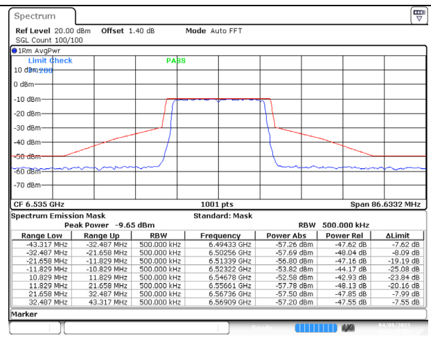
802.11ax (20MHz) 6535MHz Chain B NSS-4
