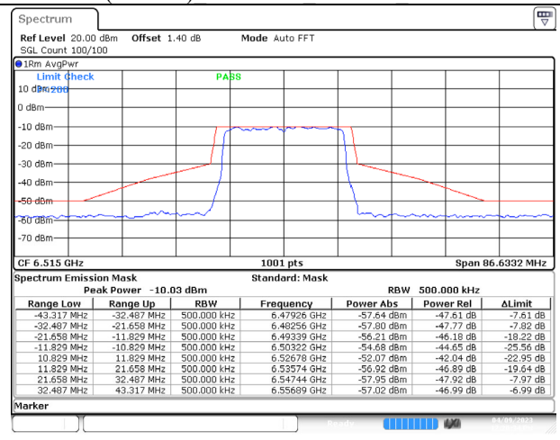
802.11ax (20MHz) 6515MHz Chain B NSS-4
