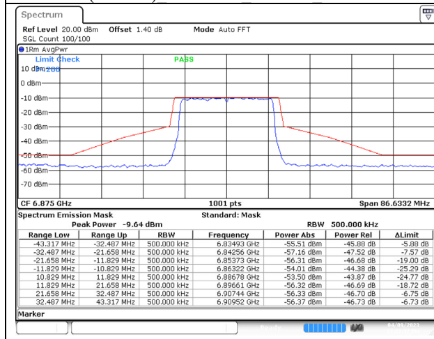
802.11ax (20MHz) 6875MHz Chain C NSS-4
