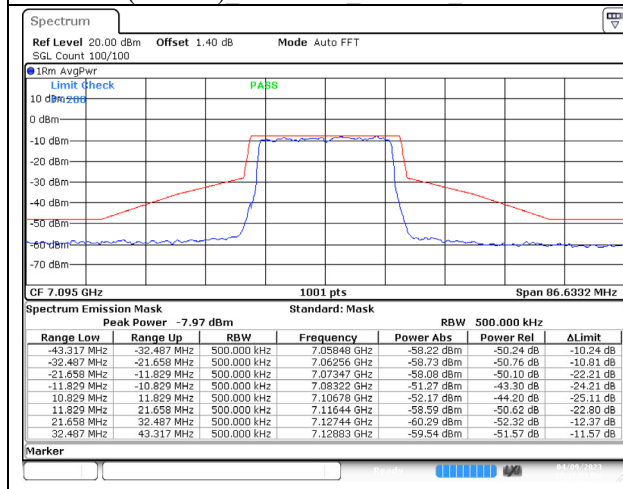
802.11ax (20MHz) 7095MHz Chain C NSS-4
