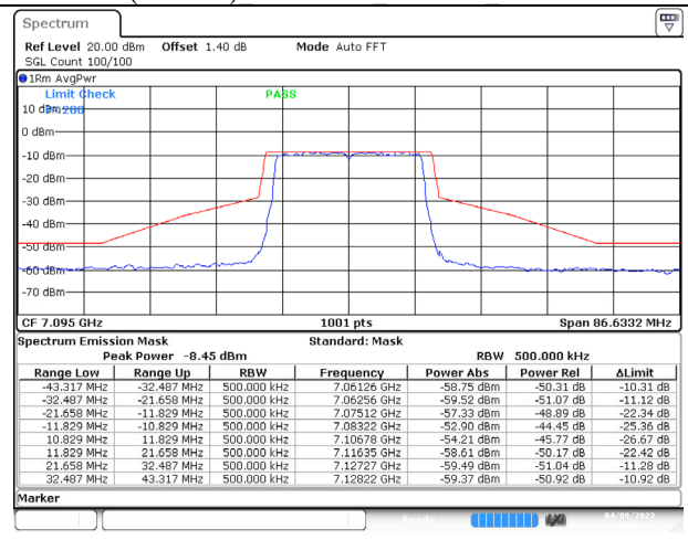
802.11ax (20MHz) 7095MHz Chain D NSS-4
