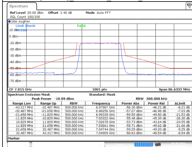
802.11ax (20MHz) 7015MHz Chain C NSS-4
