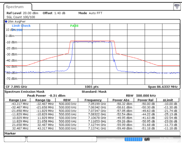
802.11ax (20MHz) 7095MHz Chain B NSS-4
