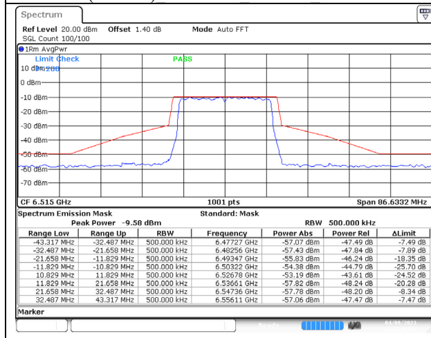
802.11ax (20MHz) 6515MHz Chain A NSS-4
