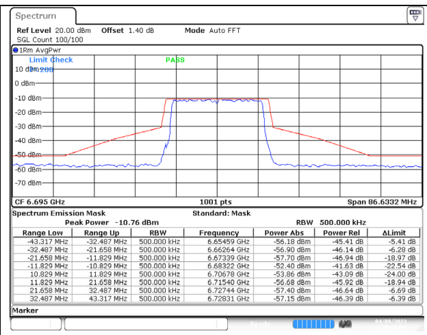
802.11ax (20MHz) 6695MHz Chain D NSS-4
