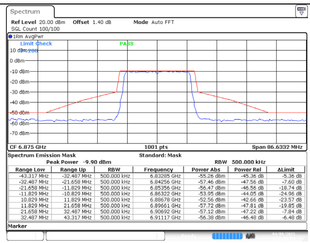
802.11ax (20MHz) 6875MHz Chain B NSS-4
