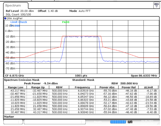
802.11ax (20MHz) 6875MHz Chain D NSS-4
