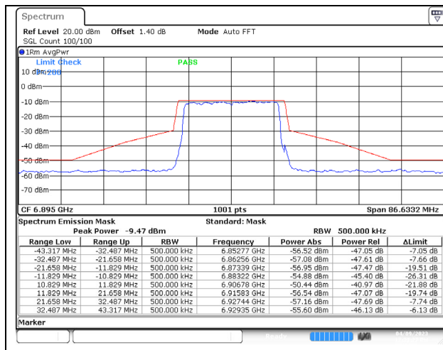
802.11ax (20MHz) 6895MHz Chain C NSS-4
