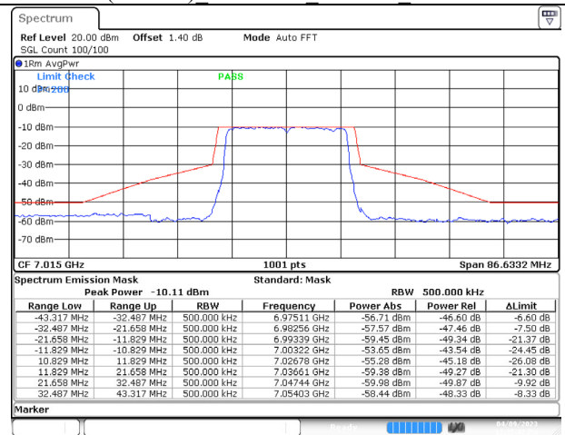
802.11ax (20MHz) 7015MHz Chain D NSS-4
