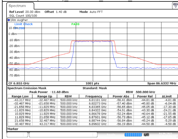
802.11ax (20MHz) 6855MHz Chain C NSS-4
