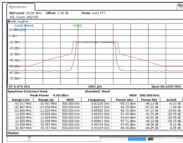
802.11ax (20MHz) 6875MHz Chain A NSS-4
