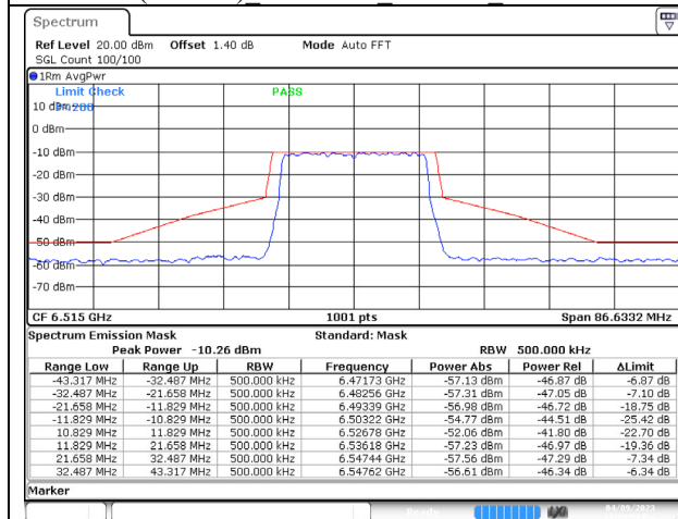
802.11ax (20MHz) 6515MHz Chain C NSS-4
