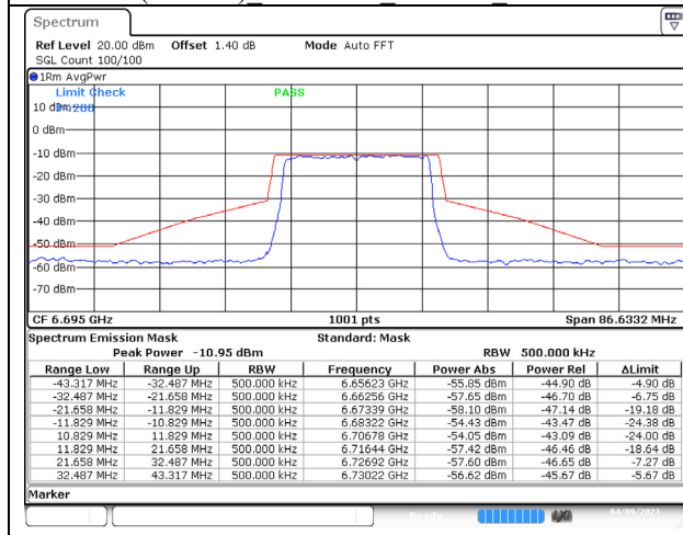
802.11ax (20MHz) 6695MHz Chain A NSS-4
