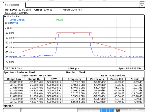
802.11ax (20MHz) 6515MHz Chain D NSS-4
