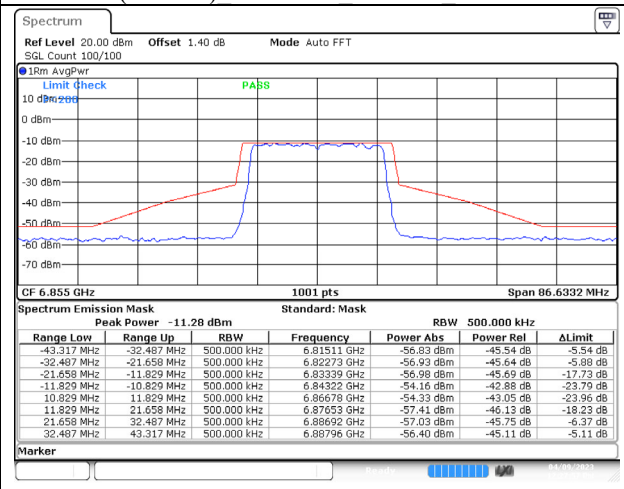
802.11ax (20MHz) 6855MHz Chain B NSS-4
