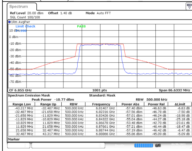
802.11ax (20MHz) 6855MHz Chain A NSS-4
