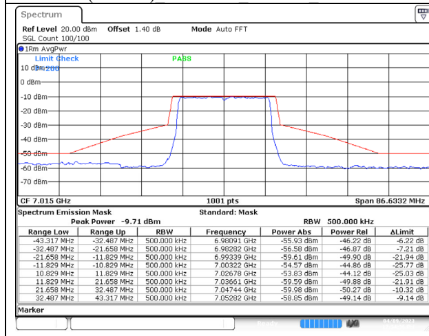
802.11ax (20MHz) 7015MHz Chain A NSS-4
