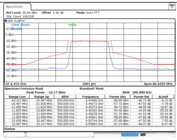
802.11ax (20MHz) 6475MHz Chain D NSS-4
