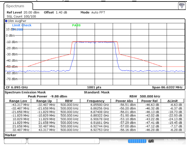
802.11ax (20MHz) 6895MHz Chain B NSS-4
