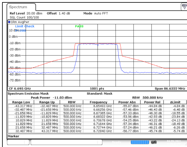
802.11ax (20MHz) 6695MHz Chain C NSS-4
