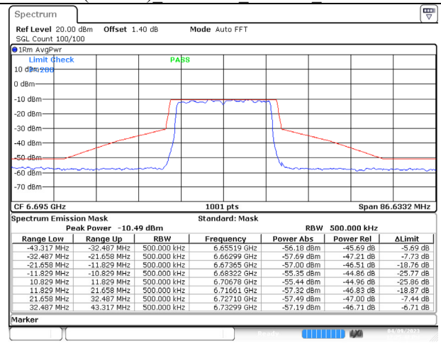
802.11ax (20MHz) 6695MHz Chain B NSS-4
