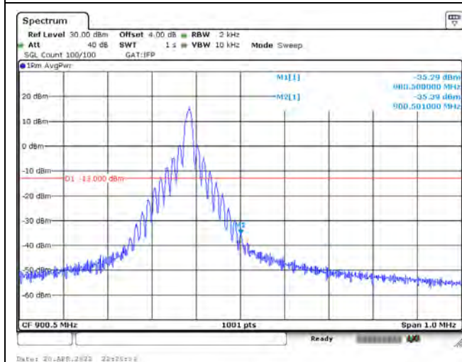
15 kHz / QPSK / CH21653 / 1RB11
