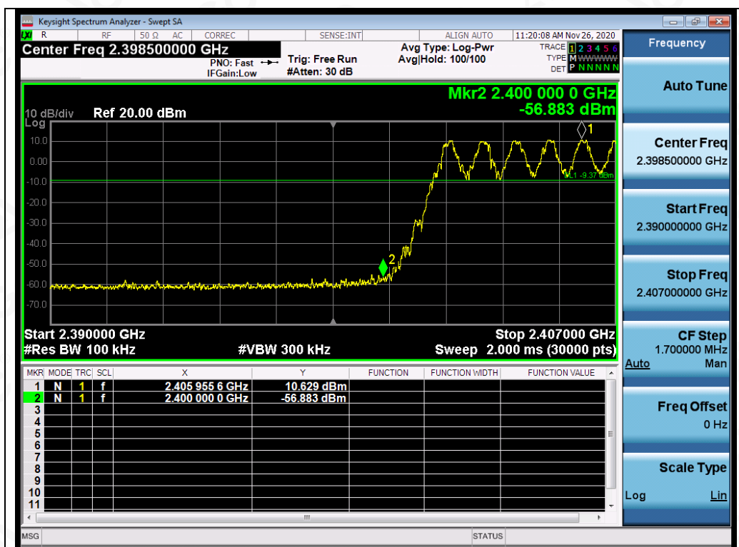
Test_Graph_BR_HOP_NA_1Mbps_Lower Band Edge Emissions
