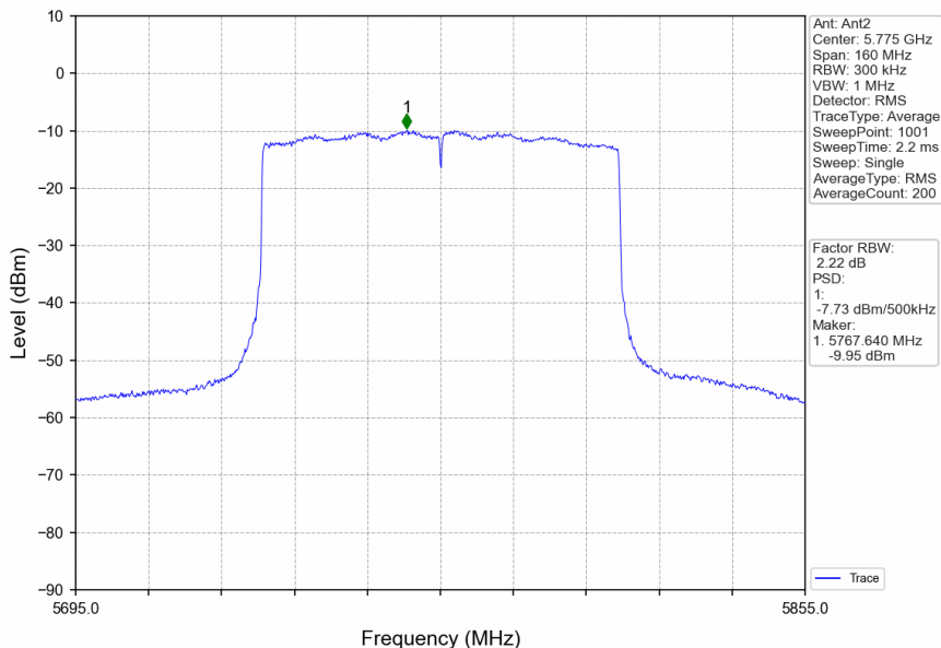
802.11ax(HEW80)_MCH_5775MHz_RU996_Left_Ant2_NTNV
