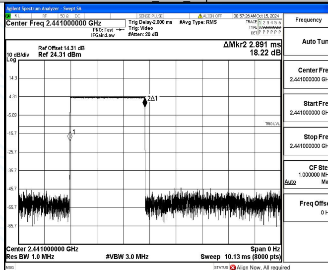
DH5_Ant1_Hop
