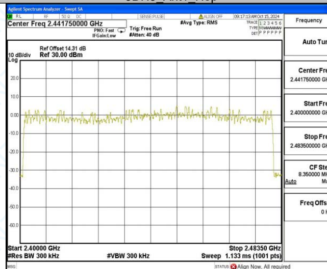
3DH5_Ant1_Hop
