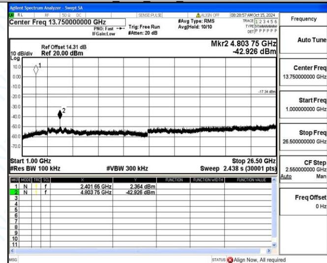
DH5_Ant1_2402_1000~26500
