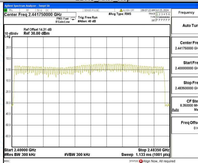
3DH5_Ant1_Hop
