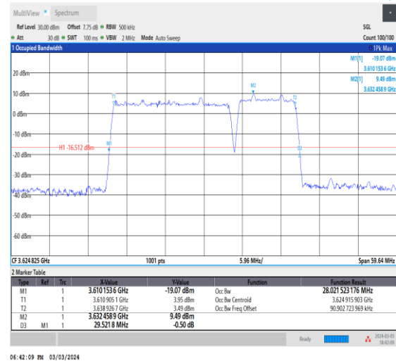
NTNV_CA_n48B_PC3_30+30_20+10_M+M_Ant0_TID2_1_#1
