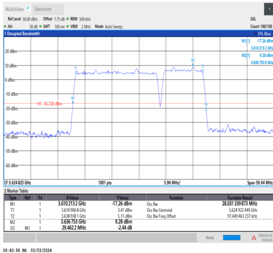
NTVN_CA_n48B_PC3_30+30_20+10_M+M_Ant0_TID9_1_#1
