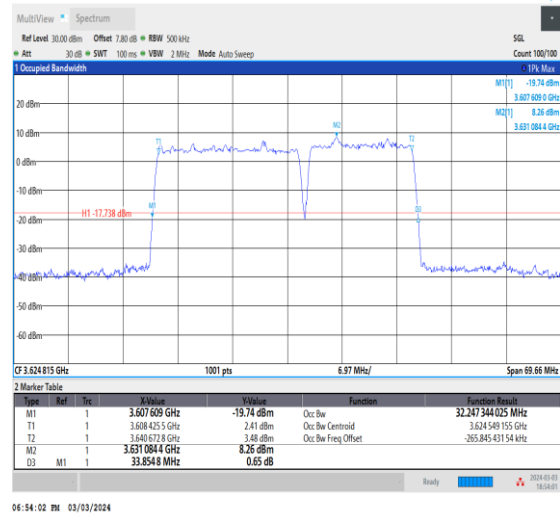
NTVN_CA_n48B_PC3_30+30_20+15_M+M_Ant0_TID1_1_#1
