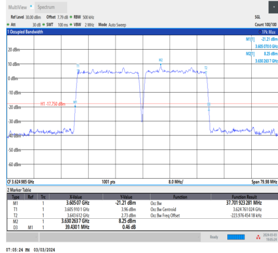
NTVN_CA_n48B_PC3_30+30_20+20_M+M_Ant0_TID2_1_#1
