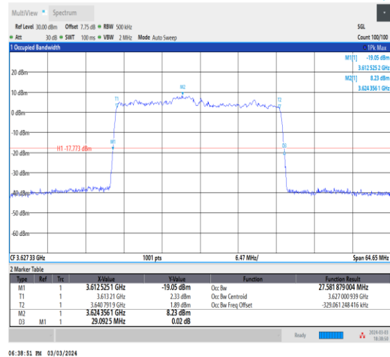
NTVN_CA_n48B_PC3_30+30_15+20_M+M_Ant0_TID7_1_#1
