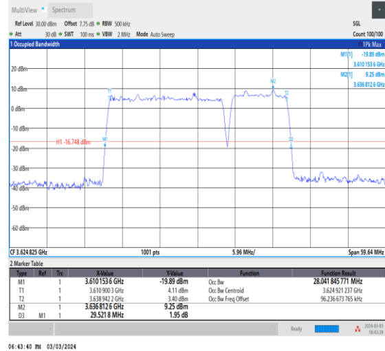
NTVN_CA_n48B_PC3_30+30_20+10_M+M_Ant0_TID8_1_#1
