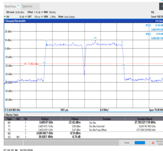
NTNV_CA_n48B_PC3_30+30_20+20_M+M_Ant0_TID6_1_#1
