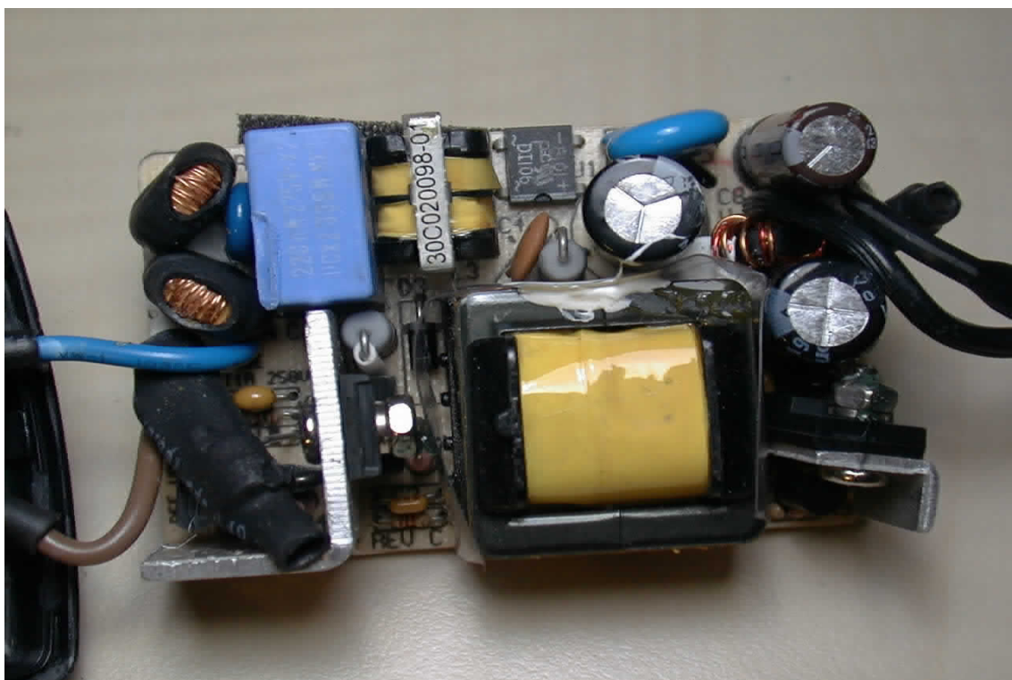
(10) EUT Photo
