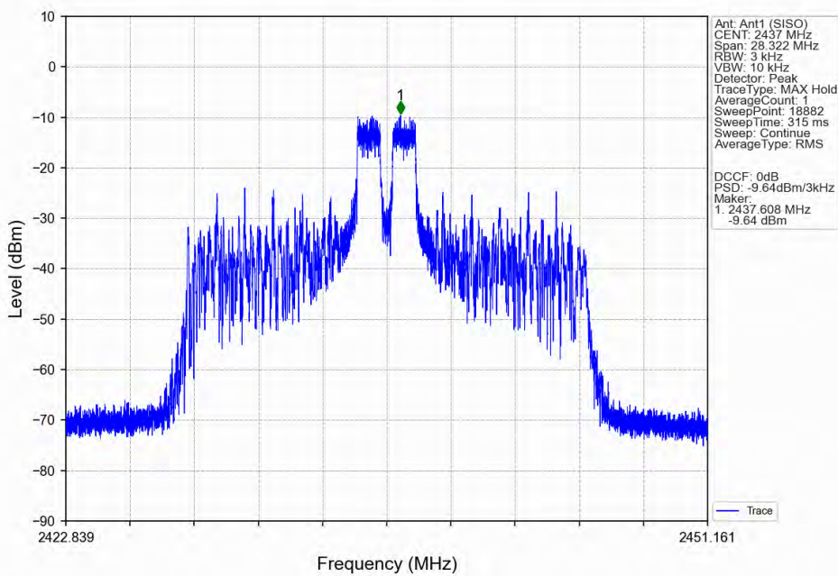
802.11ax(HEW20)_MCH_2437MHz_RU26_Left_Ant1 (SISO)_NTNV
