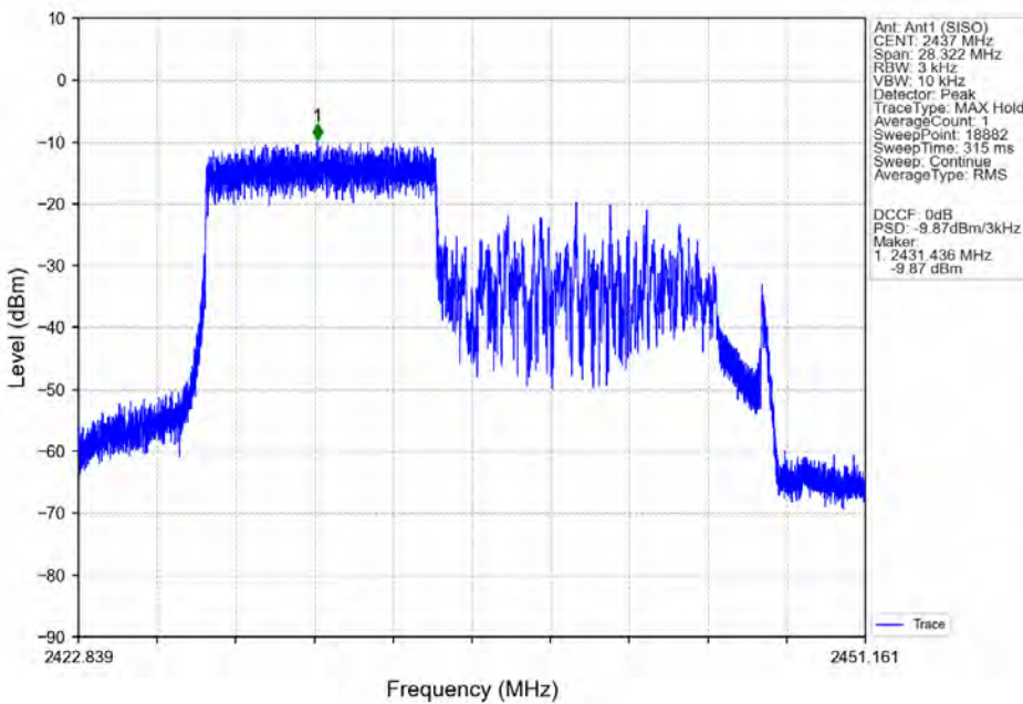
802.11ax(HEW20)_MCH_2437MHz_RU106_Left_Ant1 (SISO)_NTNV
