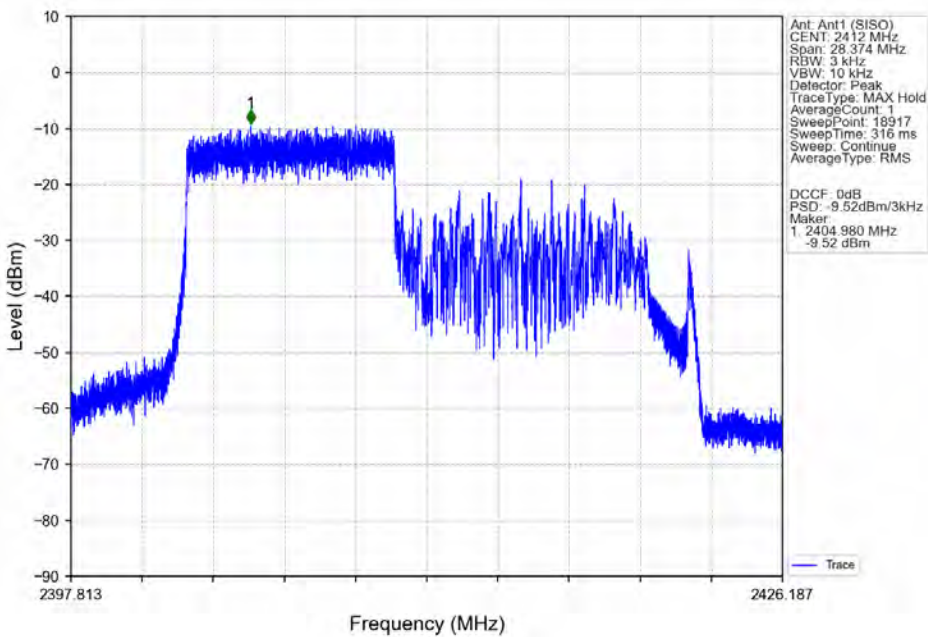
802.11ax(HEW20)_LCH_2412MHz_RU106_Left_Ant1 (SISO)_NTNV
