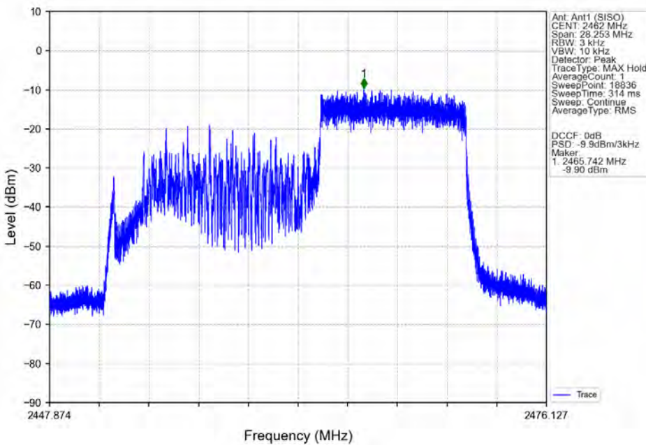
802.11ax(HEW20)_HCH_2462MHz_RU106_Left_Ant1 (SISO)_NTNV
