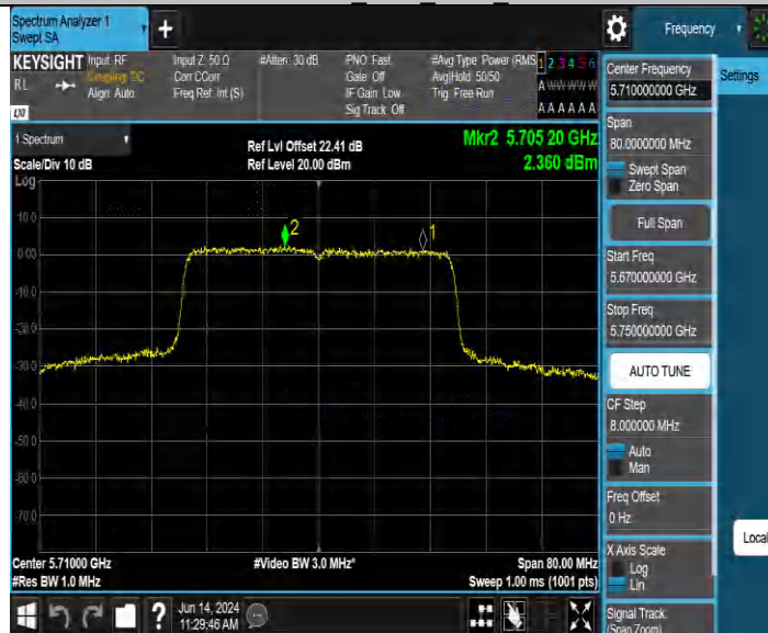
11BE40MIMO_Ant2 5710 UNII-2C
