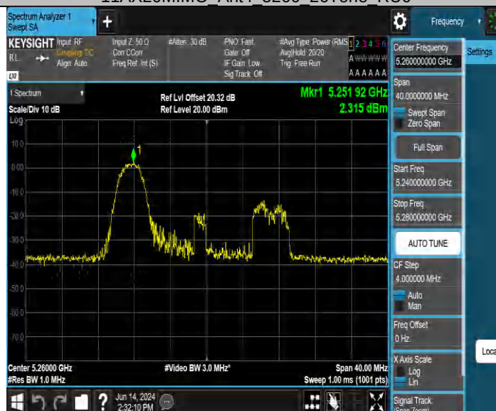
11AX20MIMO Ant4 5260 106Tone RU53
