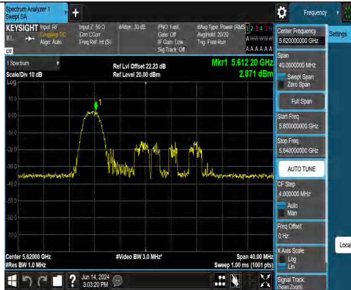
11AX20MIMO Ant1 5620 106Tone RU53
