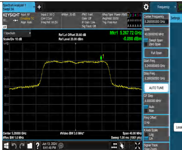
11BE20MIMO_Ant3_5260
