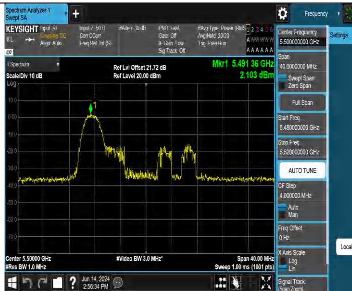
11AX20MIMO Ant2 5500 106Tone RU53
