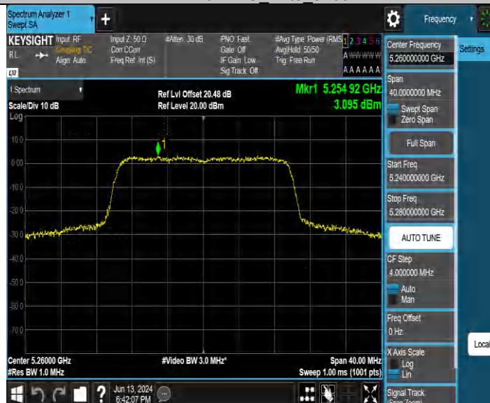
11BE20MIMO_Ant4_5260
