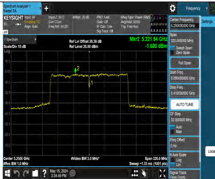
11BE160MIMO Ant4 5250 UNII-1
