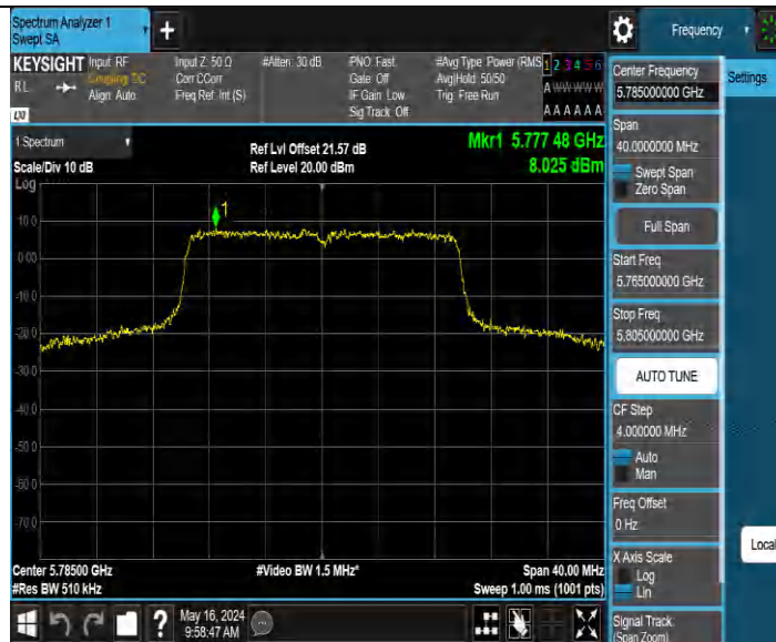
11BE20MIMO_Ant3_5785
