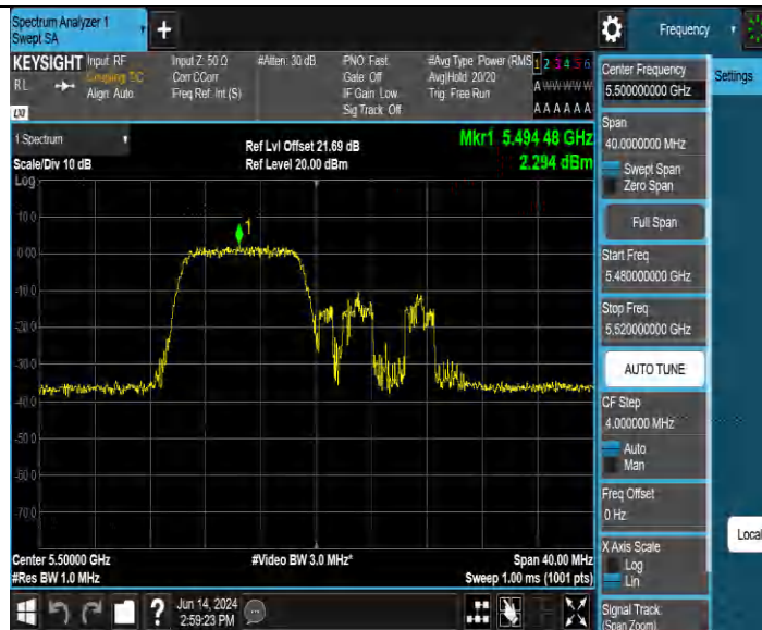
11AX20MIMO Ant4 5500 26Tone RU0
