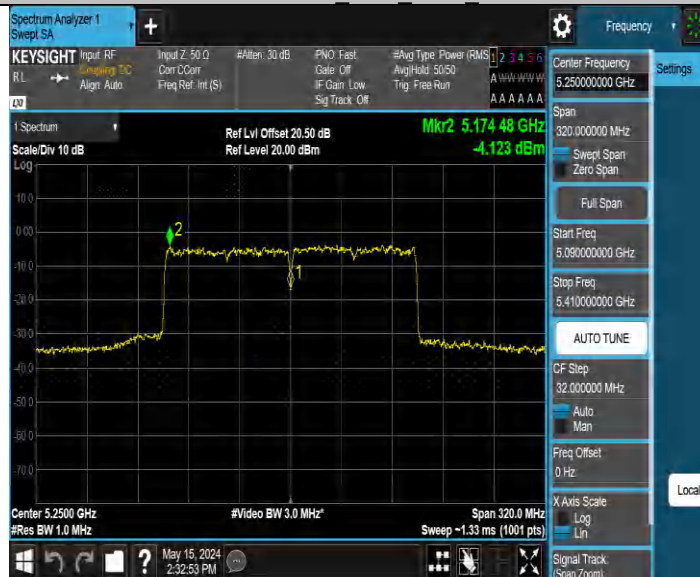
11BE160MIMO_Ant3_5250_UNII-1
