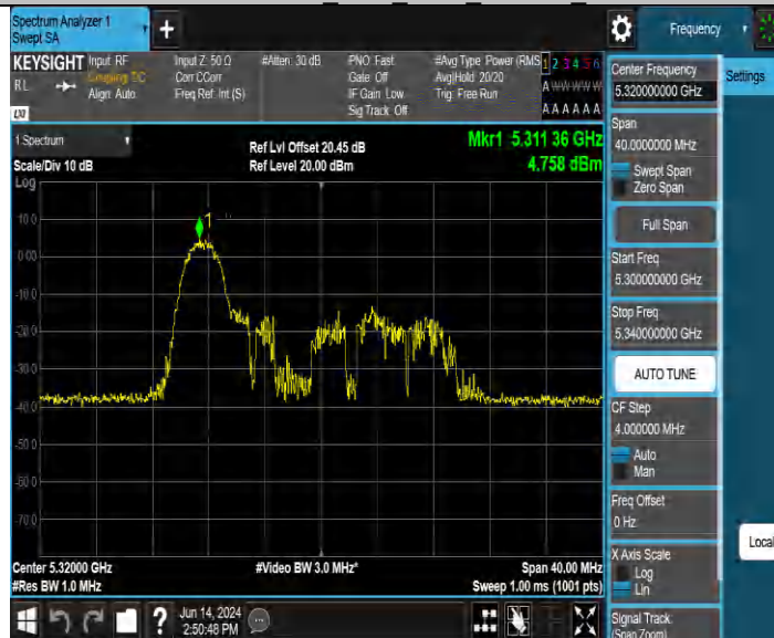
11AX20MIMO_Ant1_5320_106Tone_RU53
