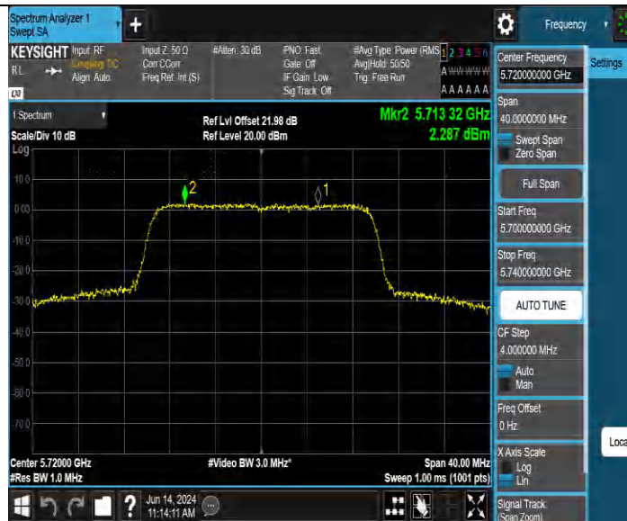
11BE20MIMO Ant3 5720 UNII-2C
