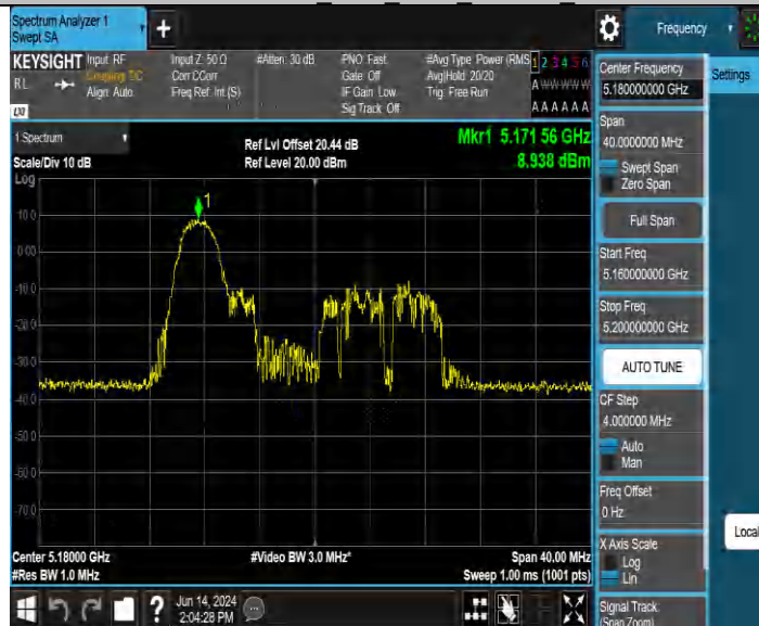
11AX20MIMO_Ant3_5180_106Tone_RU53
