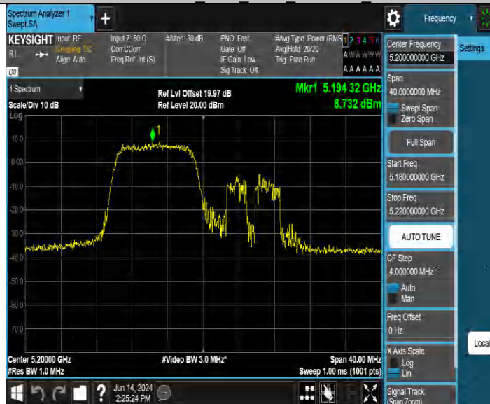
11AX20MIMO Ant4 5200 26Tone RU0
