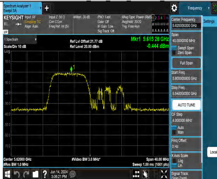
11AX20MIMO Ant4 5620 26Tone RU0
