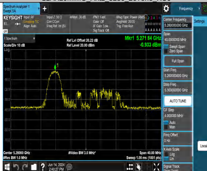
11AX20MIMO_Ant2_5280_106Tone_RU53
