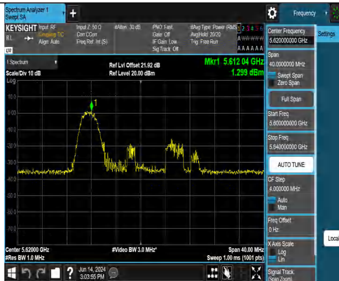
11AX20MIMO Ant4 5620 106Tone RU53
