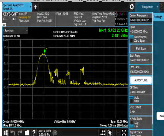
11AX20MIMO Ant3 5500 106Tone RU53
