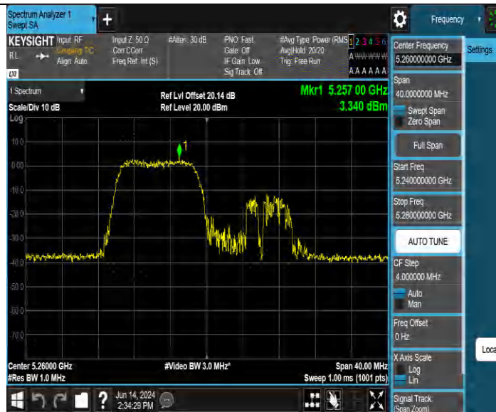
11AX20MIMO Ant4 5260 26Tone RU0
