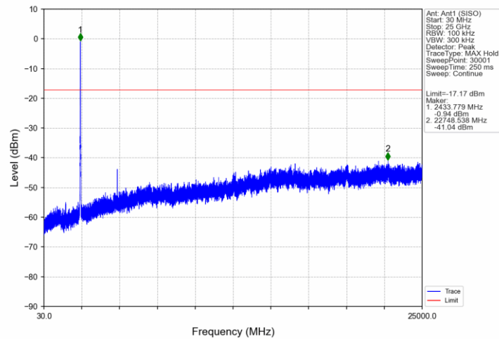
802.11n(HT40)_HCH_2452MHz_Ant1 (SISO)_NTNV
