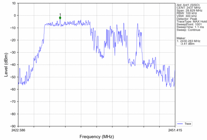
802.11ax(HEW20)_MCH_2437MHz_RU242_61_Ant1 (SISO)_NTNV
