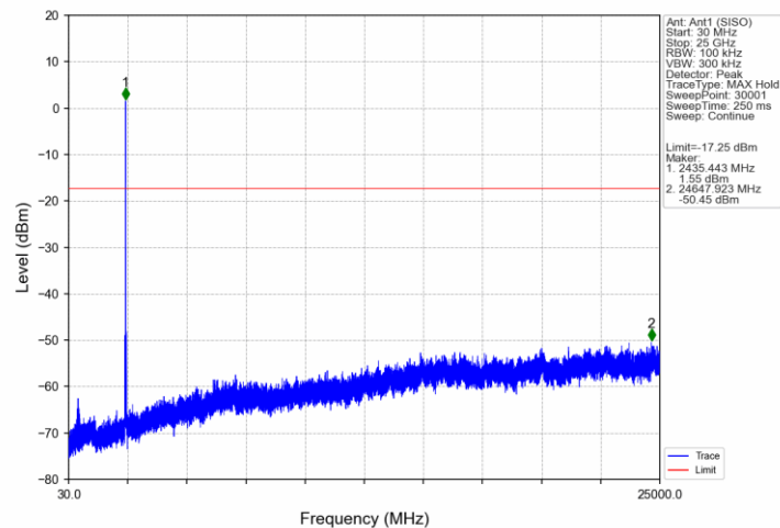
802.11ax(HEW40)_MCH_2437MHz_RU52_40_Ant1 (SISO)_NTNV
