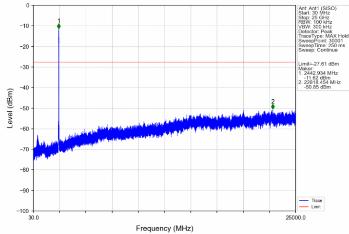
802.11ax(HEW40)_HCH_2452MHz_RU26_17_Ant1 (SISO)_NTNV
