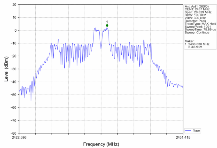
802.11ax(HEW20)_MCH_2437MHz_RU52_38_Ant1 (SISO)_NTNV
