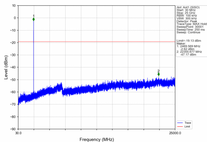
802.11ax(HEW20)_HCH_2462MHz_RU52_40_Ant1 (SISO)_NTNV
