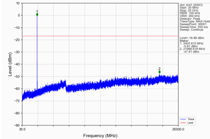
802.11ax(HEW20)_LCH_2412MHz_RU52_37_Ant1 (SISO)_NTNV
