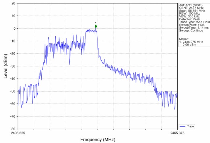
802.11ax(HEW40)_MCH_2437MHz_RU106_54_Ant1 (SISO)_NTNV
