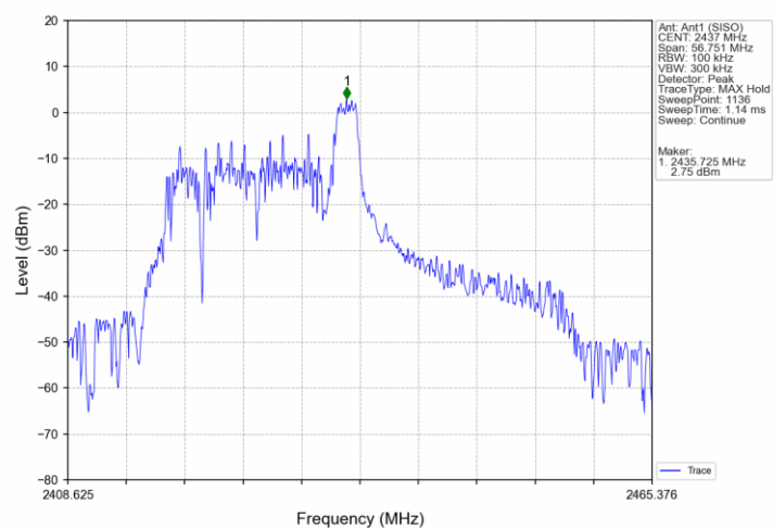
802.11ax(HEW40)_MCH_2437MHz_RU52_40_Ant1 (SISO)_NTNV
