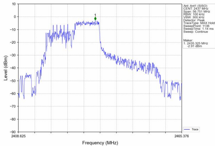
802.11ax(HEW40)_MCH_2437MHz_RU242_61_Ant1 (SISO)_NTNV
