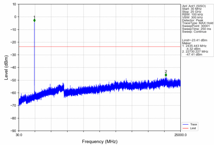
802.11ax(HEW20)_MCH_2437MHz_RU242_61_Ant1 (SISO)_NTNV
