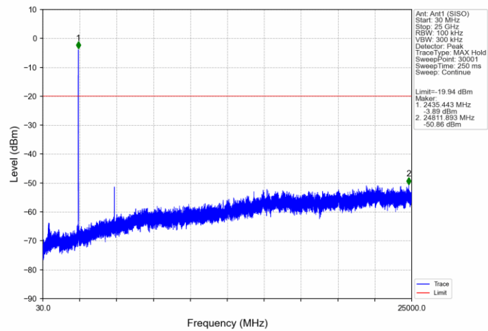
802.11ax(HEW40)_MCH_2437MHz_RU106_54_Ant1 (SISO)_NTNV
