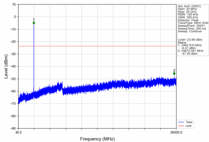
802.11ax(HEW20)_HCH_2462MHz_RU242_61_Ant1 (SISO)_NTNV
