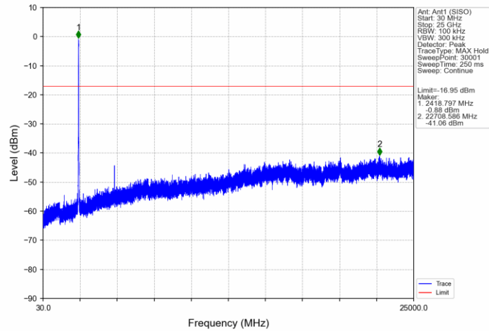
802.11n(HT40)_MCH_2437MHz_Ant1 (SISO)_NTNV
