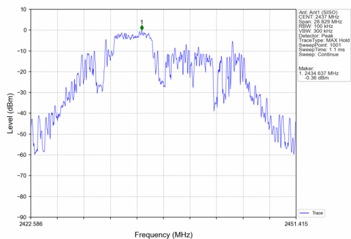
802.11ax(HEW20)_MCH_2437MHz_RU106_53_Ant1 (SISO)_NTNV
