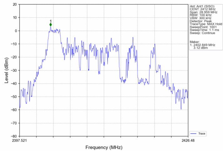
802.11ax(HEW20)_LCH_2412MHz_RU52_37_Ant1 (SISO)_NTNV
