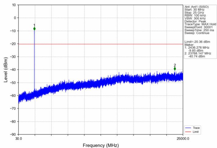
802.11ax(HEW20)_MCH_2437MHz_RU106_53_Ant1 (SISO)_NTNV
