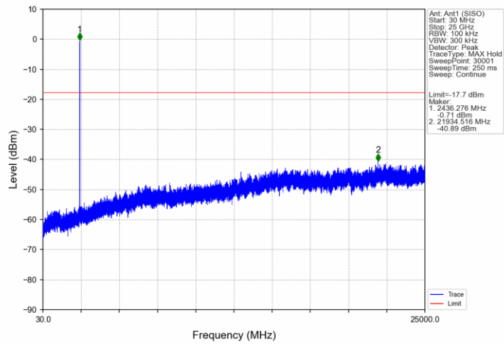
802.11ax(HEW20)_MCH_2437MHz_RU52_38_Ant1 (SISO)_NTNV
