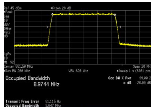
LTE10_256QAM
