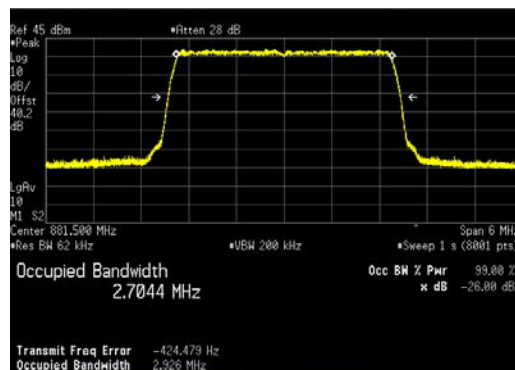
LTE3_256QAM
