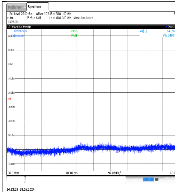
NTNV-N77-3700-3980-PC3-30-20-M-DFT-QPSK- Edge_1RB_Left-30-1000-Ant1-PASS
