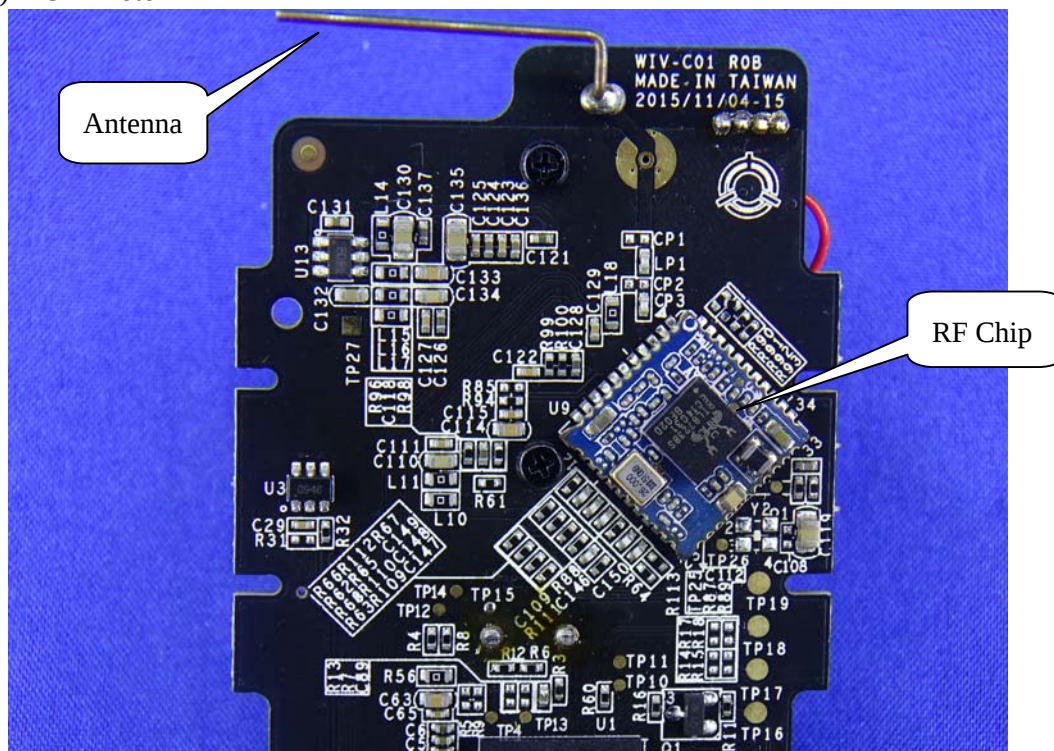
(17) EUT Photo
