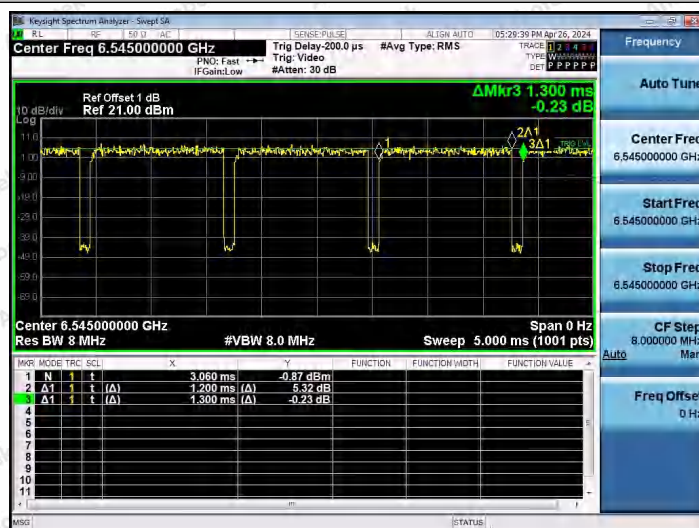
NTNV-11AX80SISO-Ant1-6545
