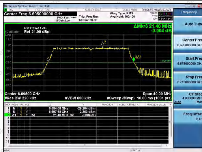
11AX20SISO-Ant1-6695
