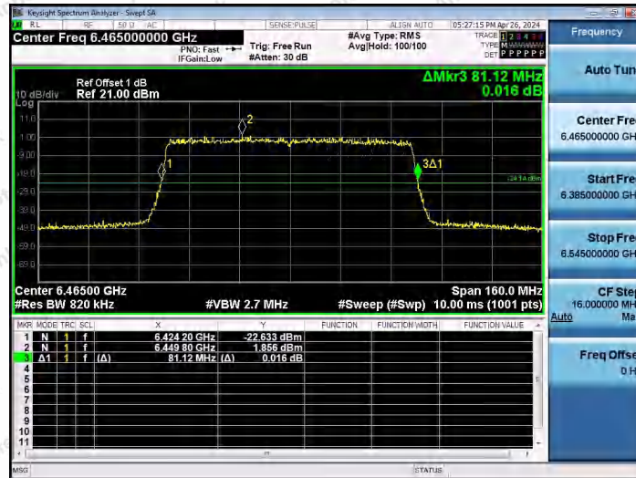
11AX80SISO-Ant1-6465
