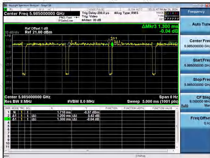
NTNV-11AX80SISO-Ant1-5985
