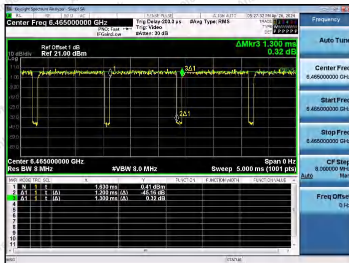
NTNV-11AX80SISO-Ant1-6465
