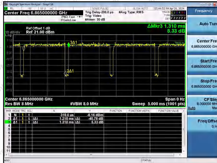
NTNV-11AX80SISO-Ant1-6865
