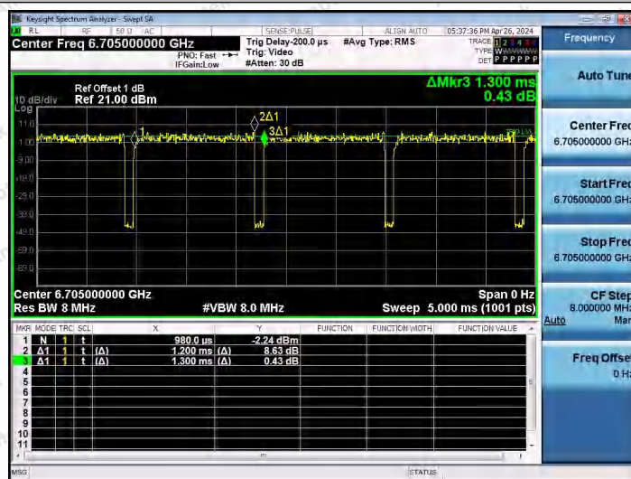
NTNV-11AX80SISO-Ant1-6705
