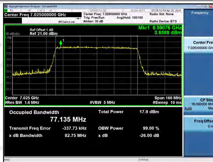
11AX80SISO-Ant1-7025-PASS
