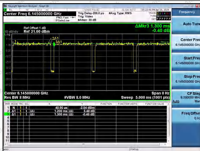
NTNV-11AX80SISO-Ant1-6145
