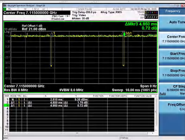
NTNV-11AX20SISO-Ant1-7115
