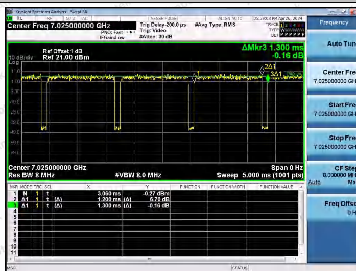
NTNV-11AX80SISO-Ant1-7025
