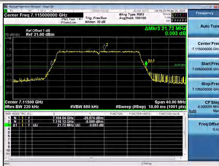
11AX20SISO-Ant1-7115
