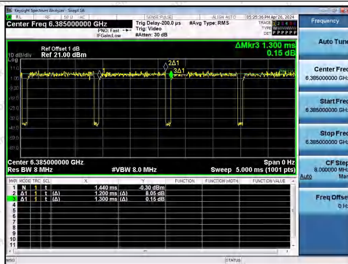
NTNV-11AX80SISO-Ant1-6385
