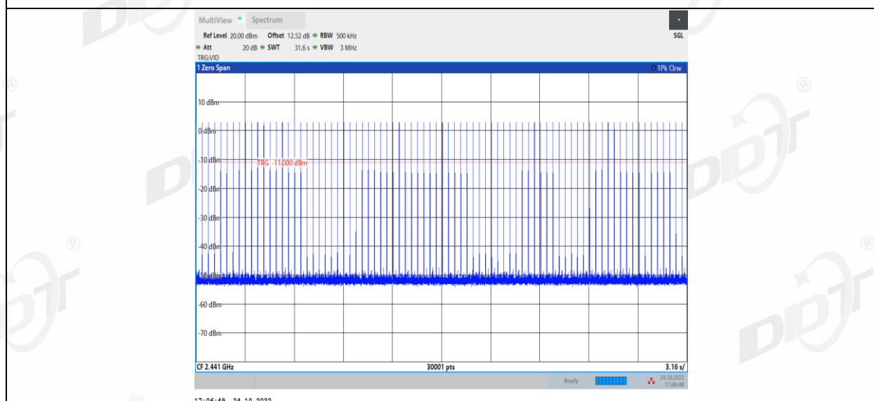
2DH3_Ant1_Hop
