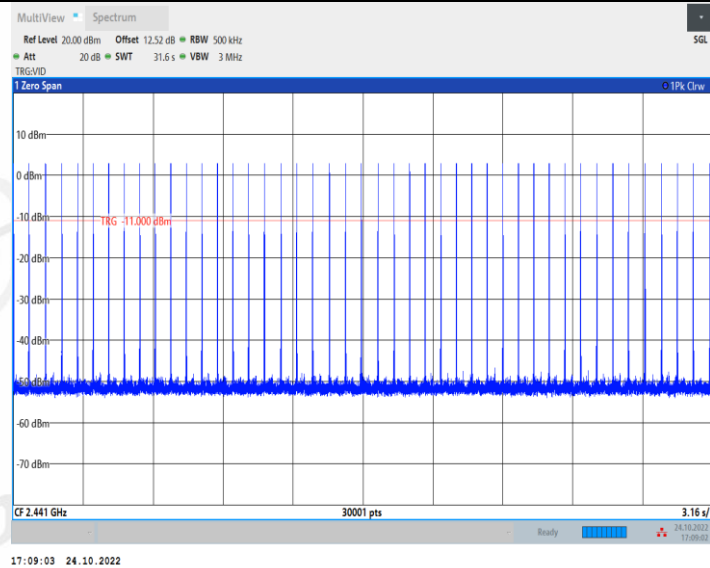
3DH1_Ant1_Hop
