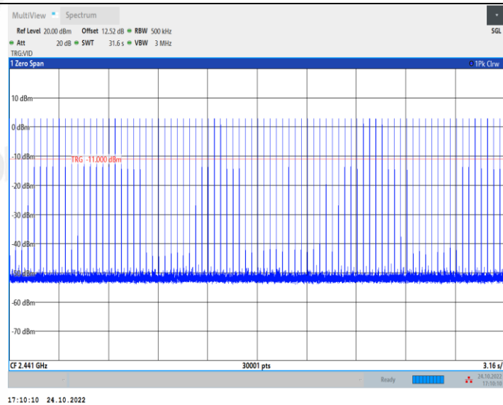
3DH3_Ant1_Hop
