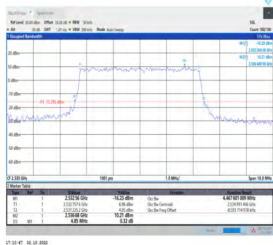
1-N7--15-5-M-7-CP-16QAM-Outer_Full-25@0-Ant1- 4.468-4.850≤5-PASS
