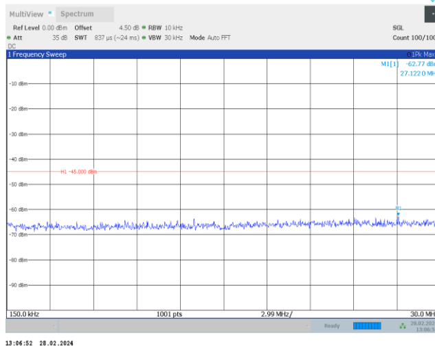
Band38-20MHz-QPSK-37850-1RB#0-Range2:0.15~30MHz
