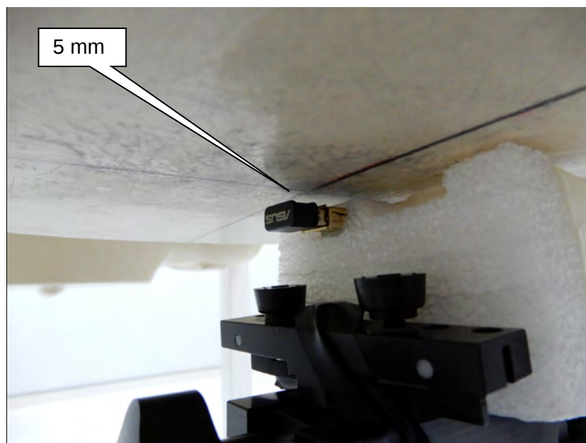
EUT Back
