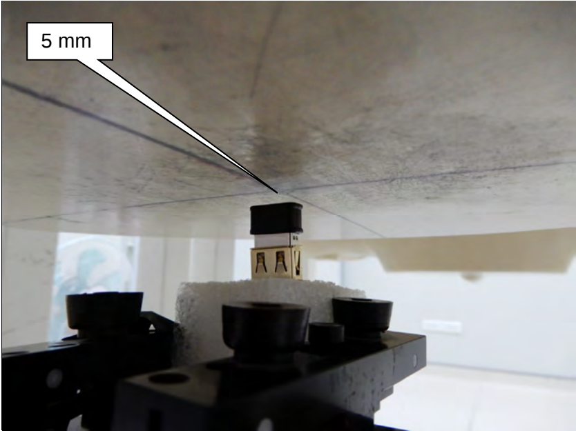
EUT Tip
