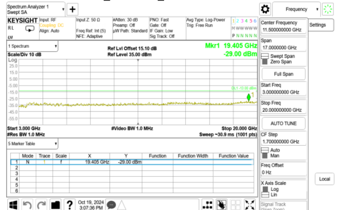
GPRS_1900MHz_MidCH661-1880
