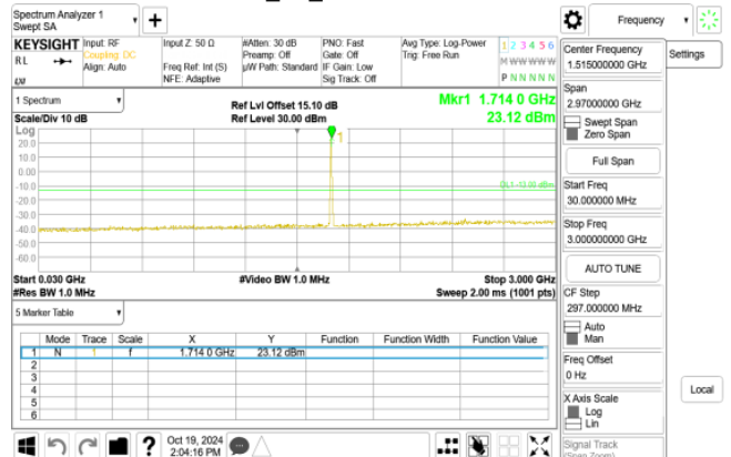
WCDMA_B4_LowCH1312-1712.4
