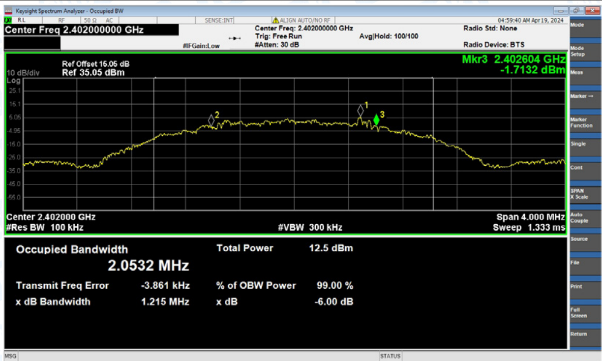
-6dB Bandwidth NVNT BLE 2Mbps 2402MHz Ant1
