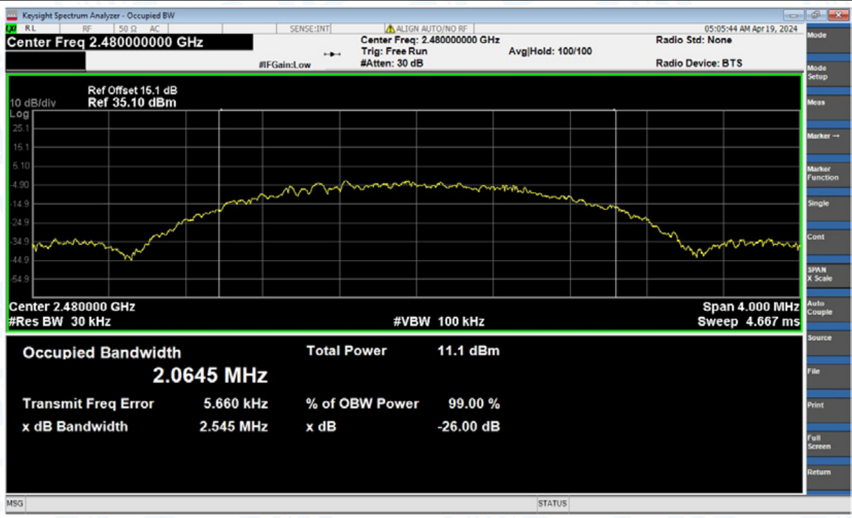
OBW NVNT BLE 2Mbps 2480MHz Ant1
