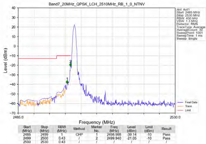
Band7_20MHz_QPSK_LCH_2510MHz_RB_1_0_NTNV
