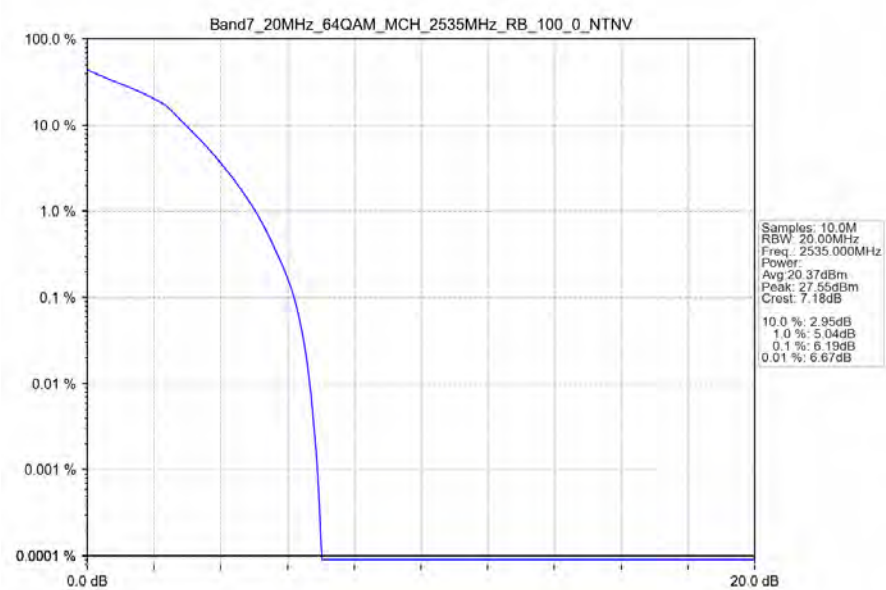
Band7_20MHz_64QAM_MCH_2535MHz_RB_100_0_NTNV
