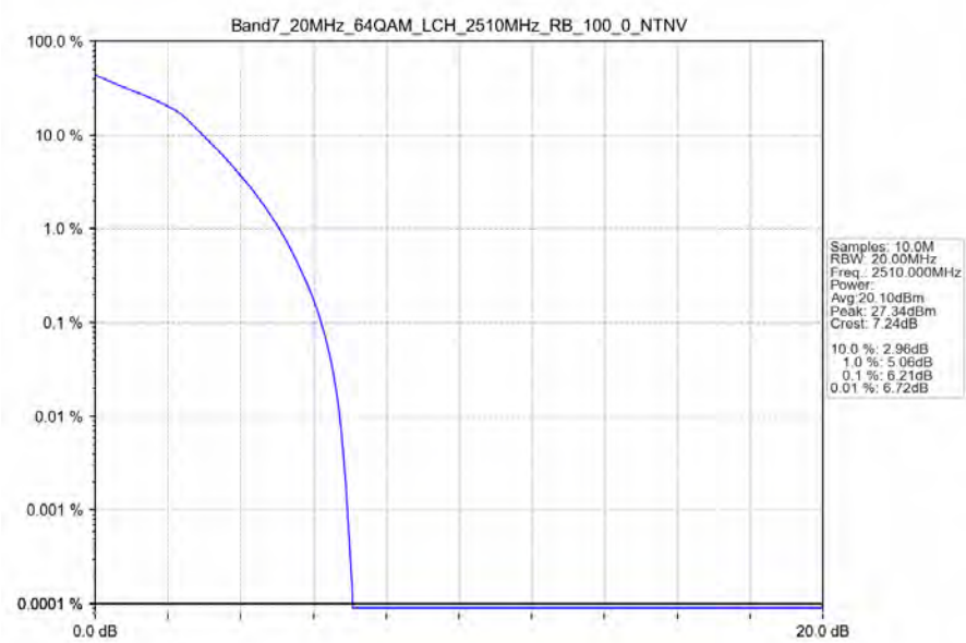
Band7_20MHz_64QAM_LCH_2510MHz_RB_100_0_NTNV
