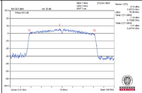
802.11ac (80MHz)_Chain 0 / CH 42
