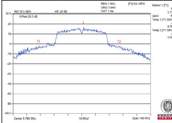
802.11ac (40MHz)_Chain 0 / CH 159
