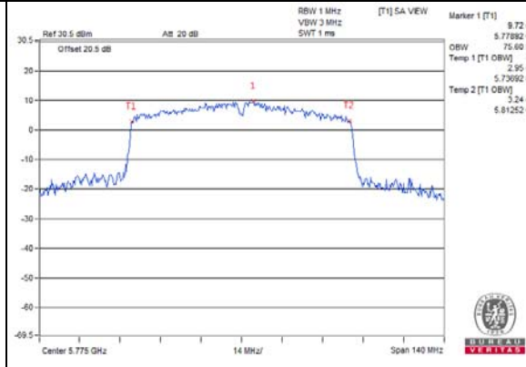
802.11ac (80MHz)_Chain 1 / CH 155
