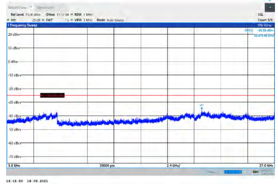
CA_38C-20MHz-20MHz-16QAM-16QAM-37901-38099-1RB#99-1RB#0-3000~27000MHz
