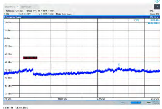
CA_7C-20MHz-20MHz-QPSK-QPSK-20850-21048-1RB#99-1RB#0-3000~27000MHz
