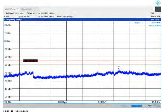
CA_38C-20MHz-20MHz-QPSK-QPSK-37850-38048-1RB#0-0RB#0-3000~27000MHz
