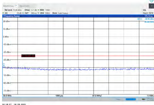
CA_38C-20MHz-20MHz-QPSK-QPSK-37850-38048-1RB#0-0RB#0-30~1000MHz
