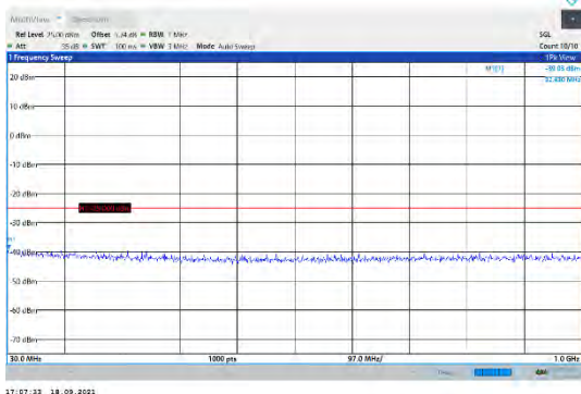
CA_41C-20MHz-20MHz-QPSK-QPSK-41292-41490-1RB#0-0RB#0-30~1000MHz
