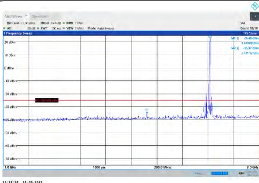
CA_38C-20MHz-20MHz-QPSK-QPSK-37901-38099-0RB#0-1RB#99-1000~3000MHz
