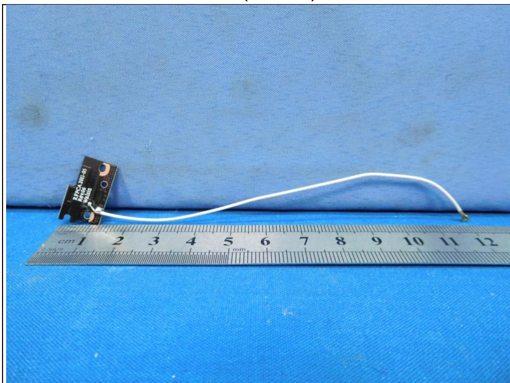
Ant 1 (WiFi+BT)
