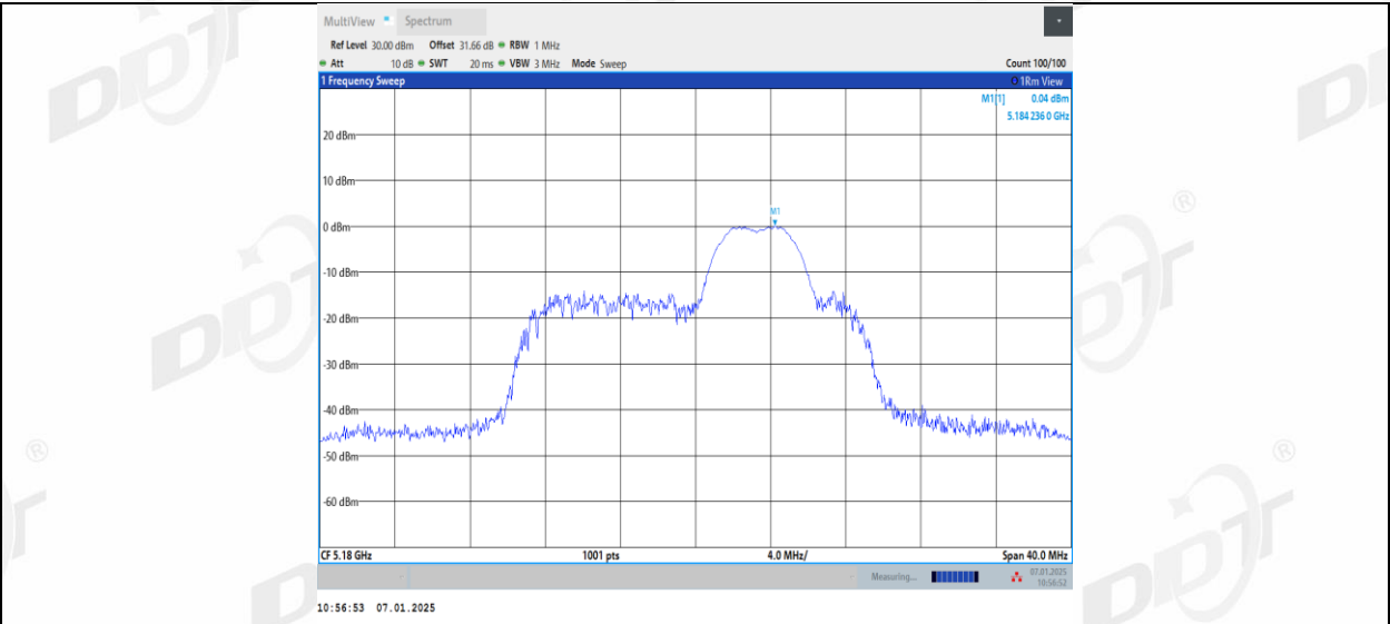
11AX20MIMO_Ant2_5180_52Tone_RU40
