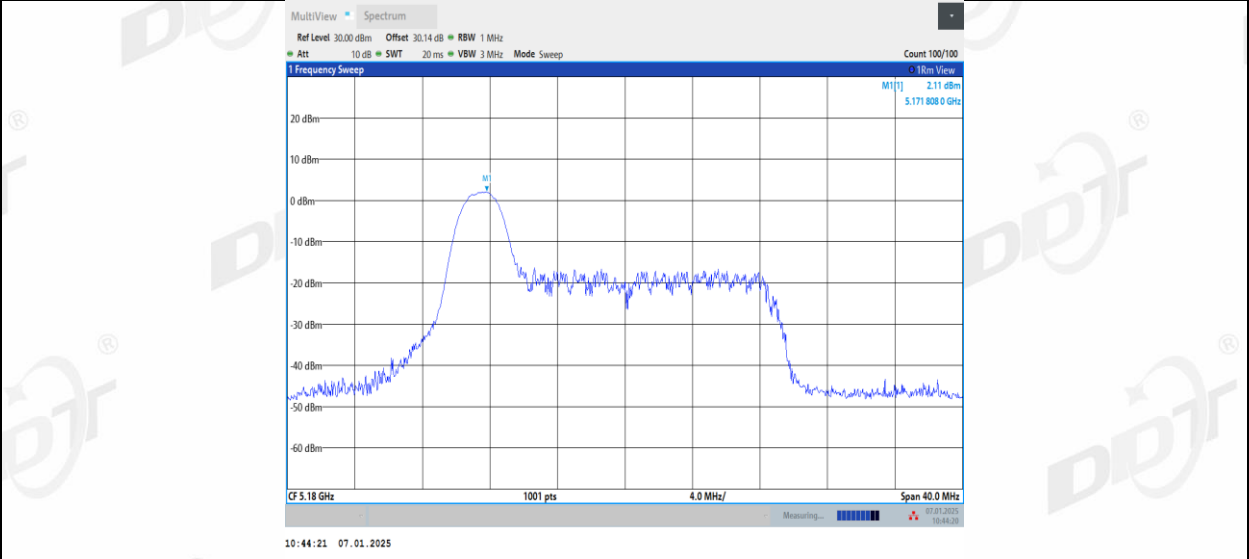
11AX20MIMO_Ant2_5180_26Tone_RU4
