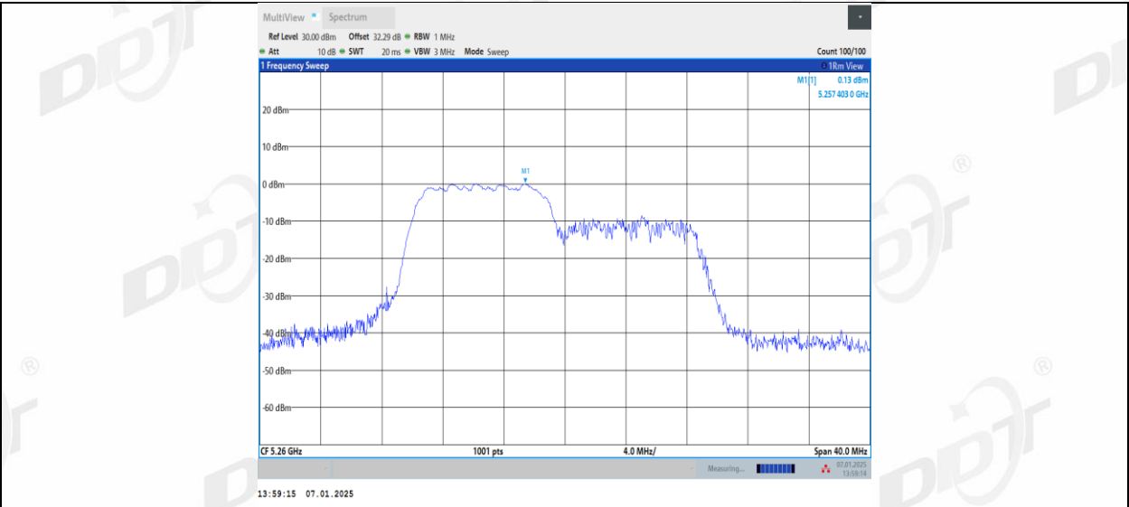
11AX20MIMO_Ant1_5260_106Tone_RU54
