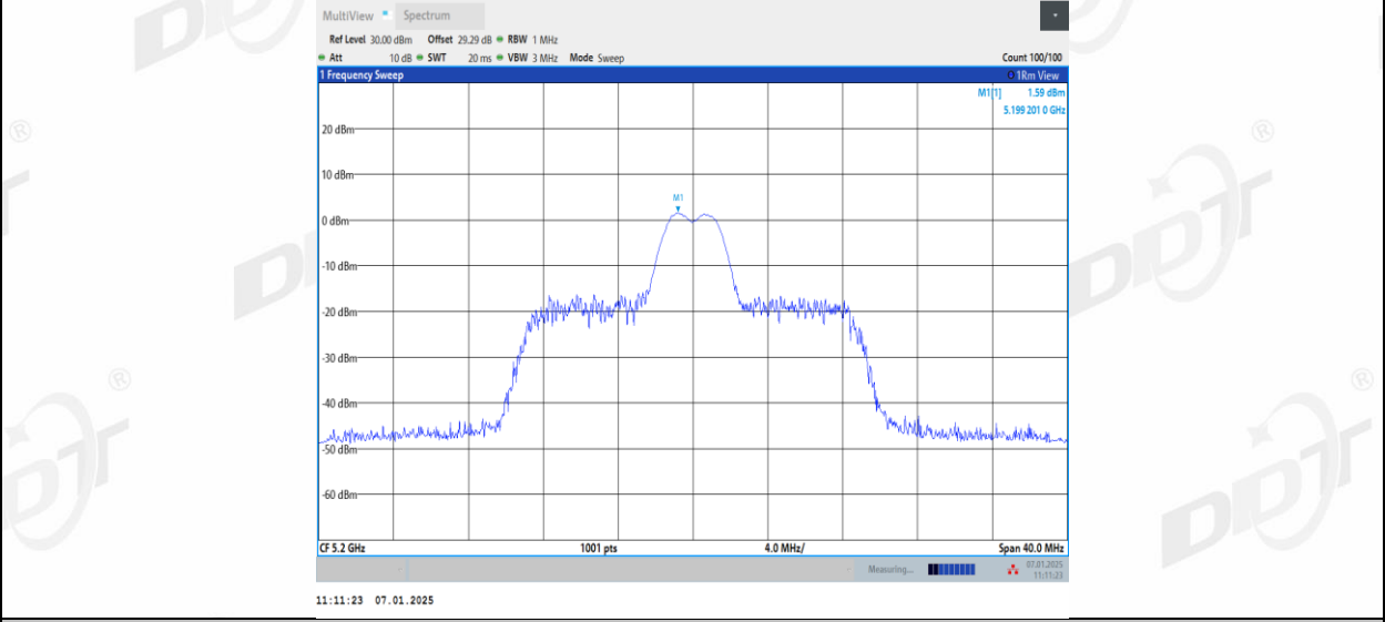
11AX20MIMO_Ant1_5200_26Tone_RU8
