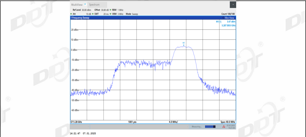
11AX20MIMO_Ant1_5280_106Tone_RU53
