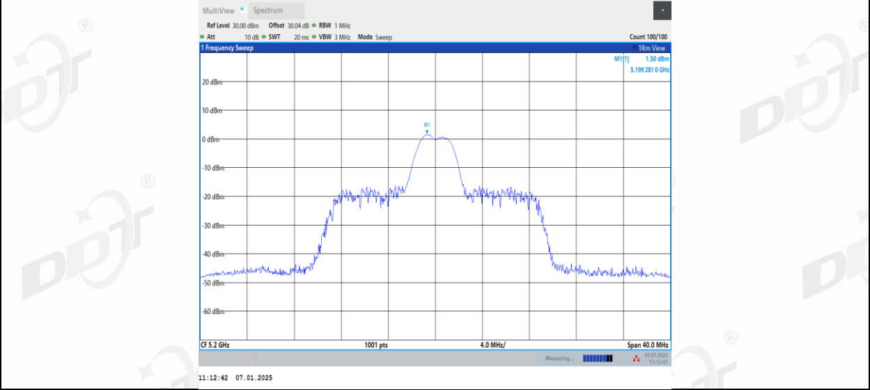
11AX20MIMO_Ant2_5200_26Tone_RU8
