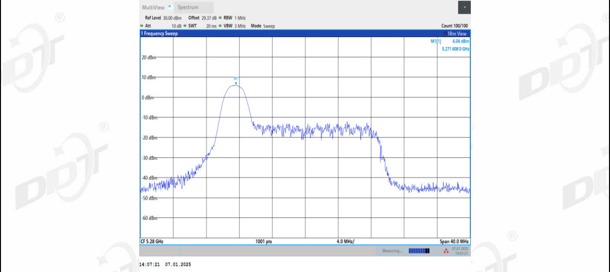
11AX20MIMO_Ant1_5280_26Tone_RU4
