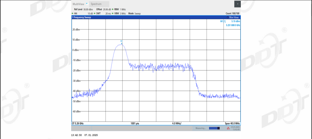
11AX20MIMO_Ant2_5260_26Tone_RU4
