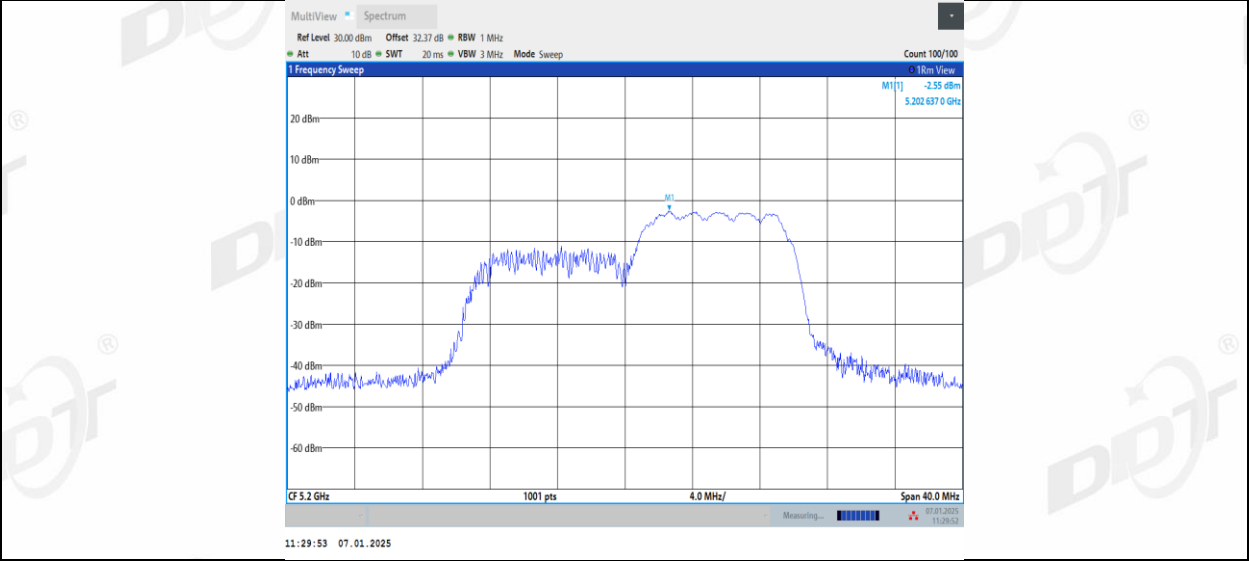
11AX20MIMO_Ant2_5200_26Tone_RU0
