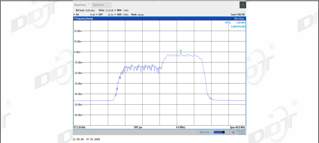
11AX20MIMO_Ant2_5240_26Tone_RU0
