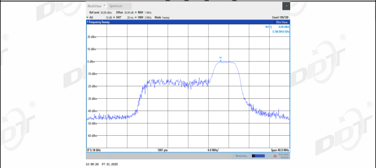
11AX20MIMO_Ant1_5180_106Tone_RU53
