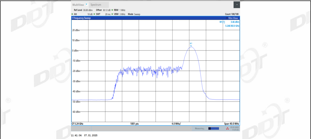
11AX20MIMO_Ant2_5240_52Tone_RU37
