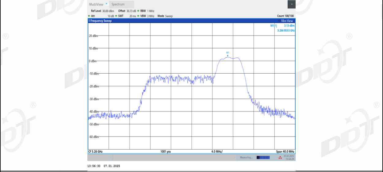
11AX20MIMO_Ant1_5260_106Tone_RU53
