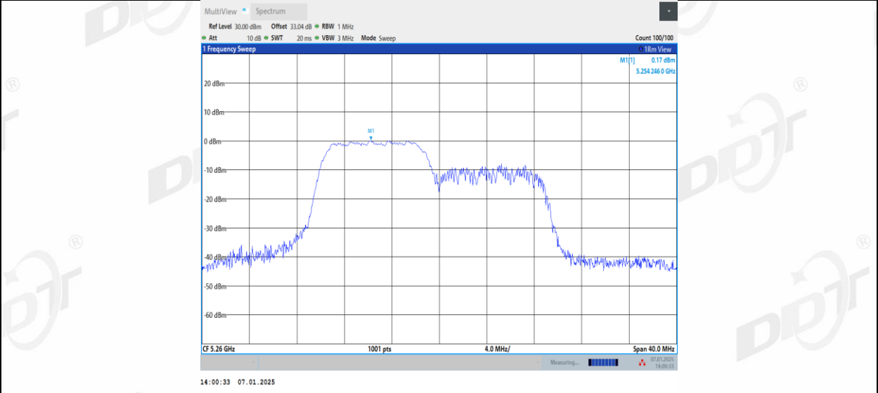
11AX20MIMO_Ant2_5260_106Tone_RU54
