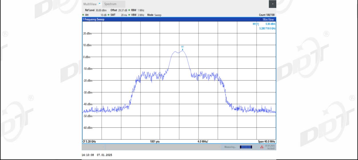
11AX20MIMO_Ant1_5280_26Tone_RU8
