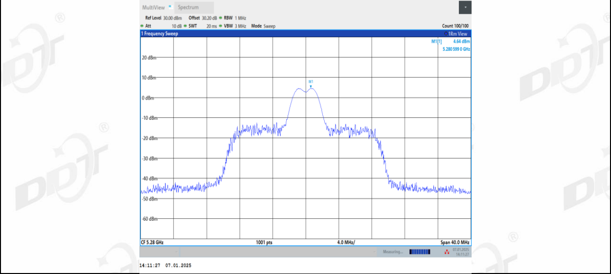
11AX20MIMO_Ant2_5280_26Tone_RU8
