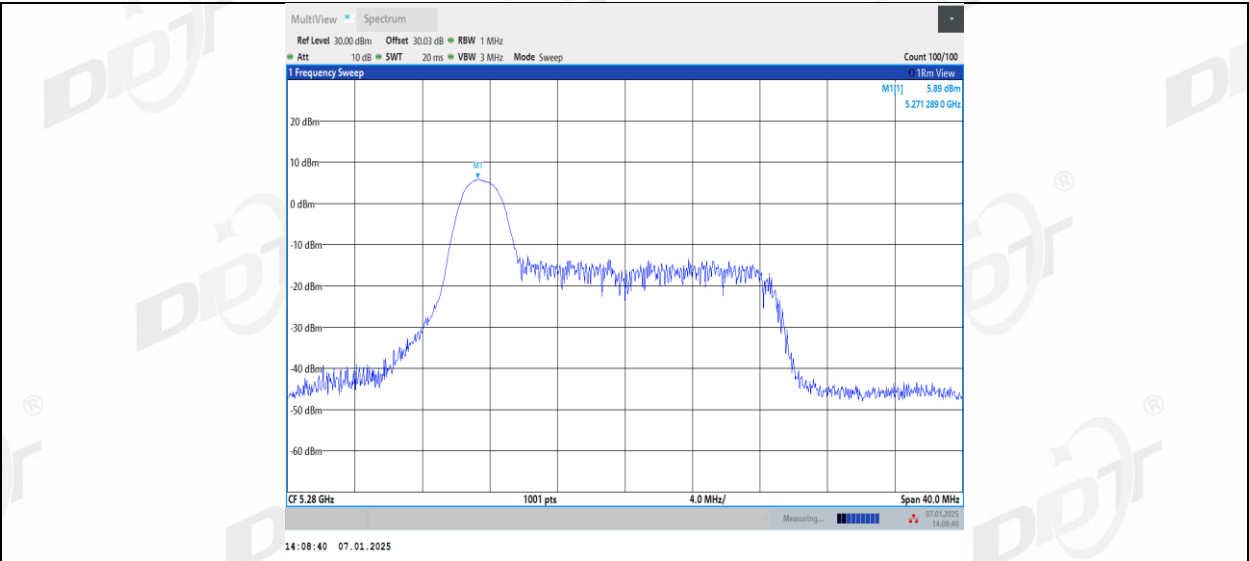
11AX20MIMO_Ant2_5280_26Tone_RU4
