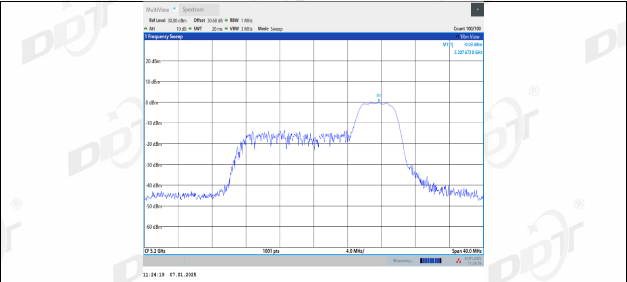
11AX20MIMO_Ant1_5200_106Tone_RU53
