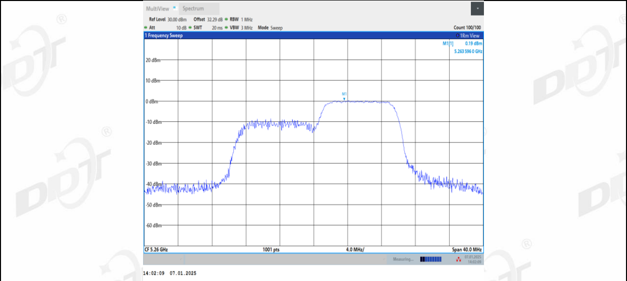
11AX20MIMO_Ant2_5260_26Tone_RU0
