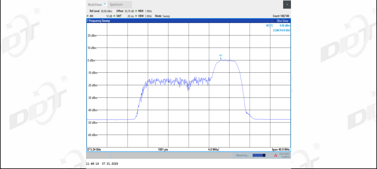
11AX20MIMO_Ant1_5240_106Tone_RU53
