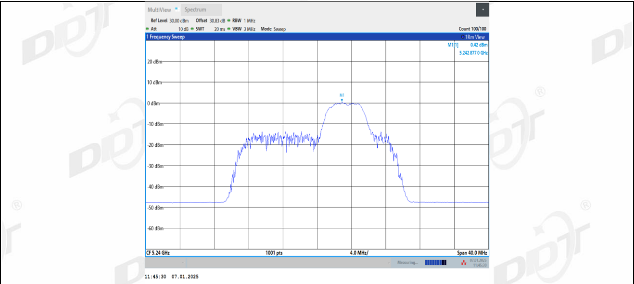
11AX20MIMO_Ant1_5240_52Tone_RU40
