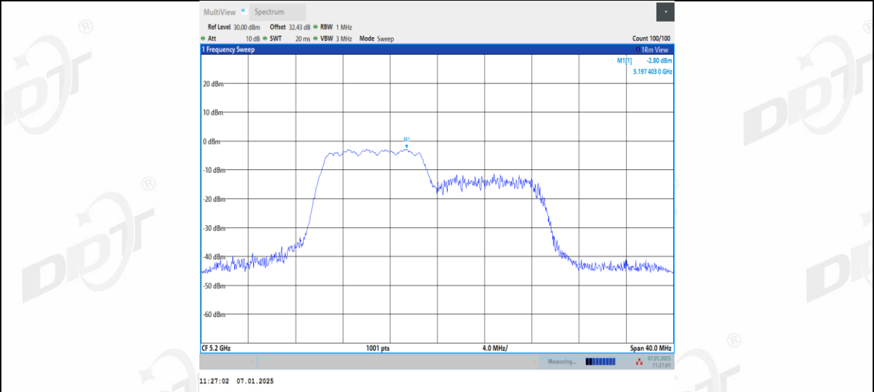
11AX20MIMO_Ant1_5200_106Tone_RU54
