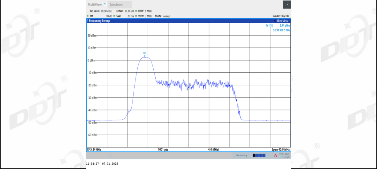
11AX20MIMO_Ant2_5240_26Tone_RU4
