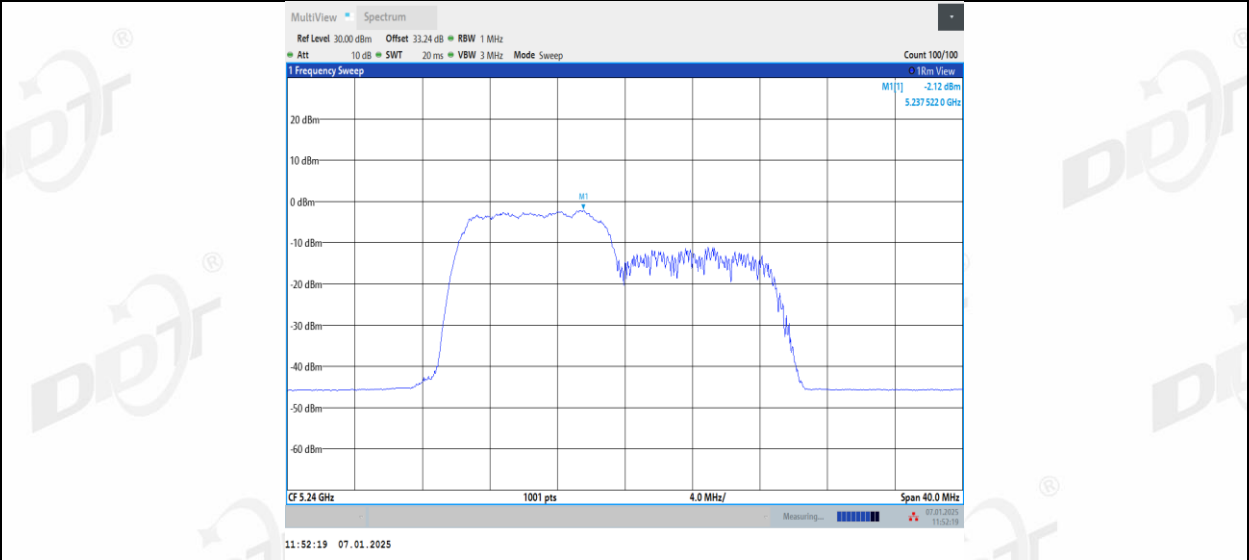
11AX20MIMO_Ant2_5240_106Tone_RU54
