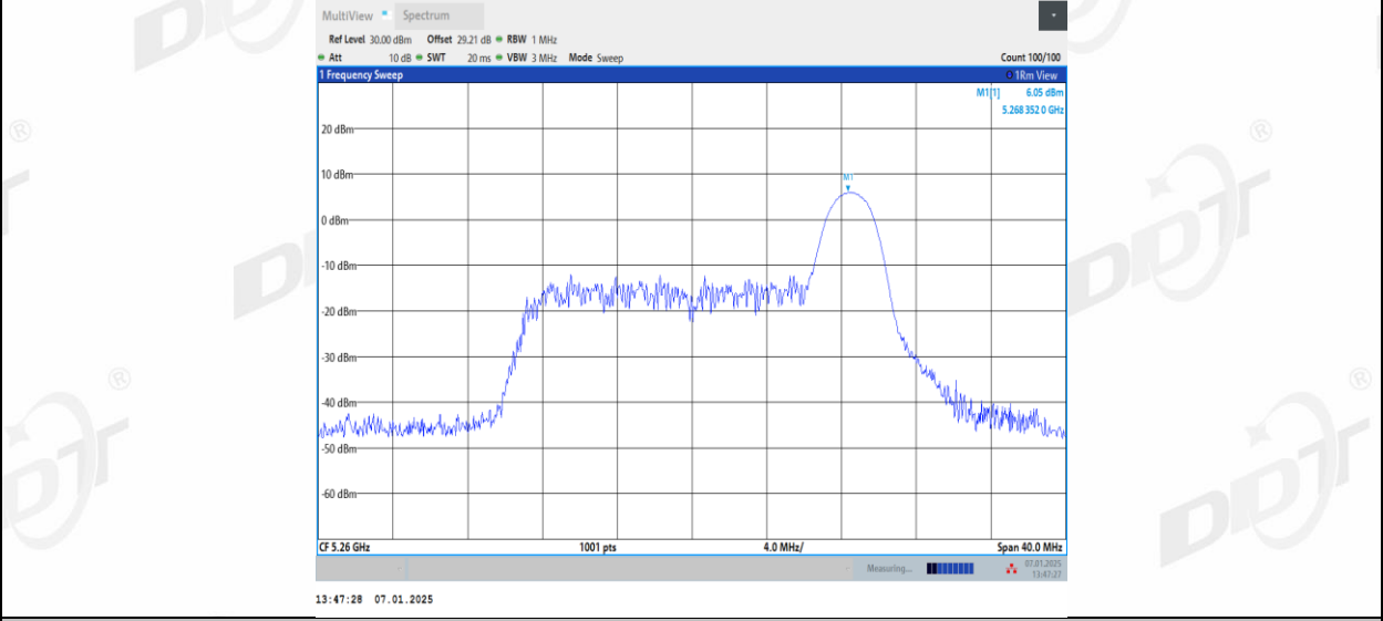
11AX20MIMO_Ant1_5260_52Tone_RU37
