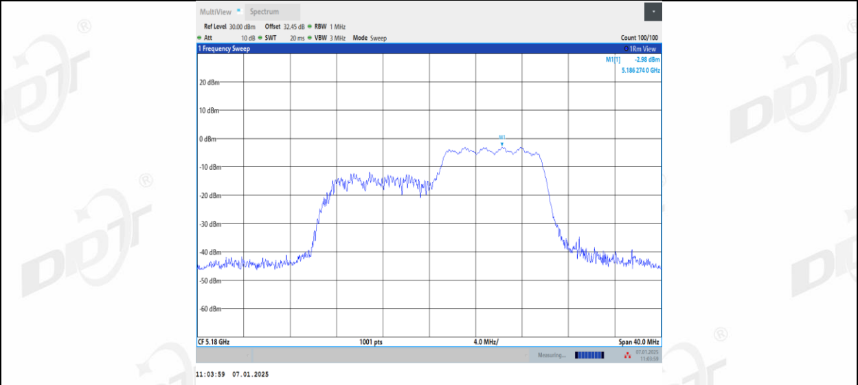
11AX20MIMO_Ant2_5180_26Tone_RU0
