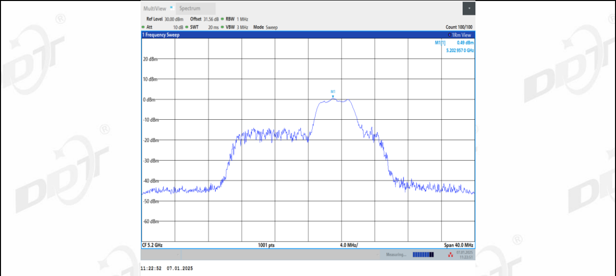
11AX20MIMO_Ant2_5200_52Tone_RU40
