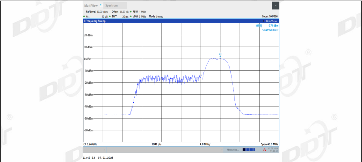
11AX20MIMO_Ant2_5240_106Tone_RU53
