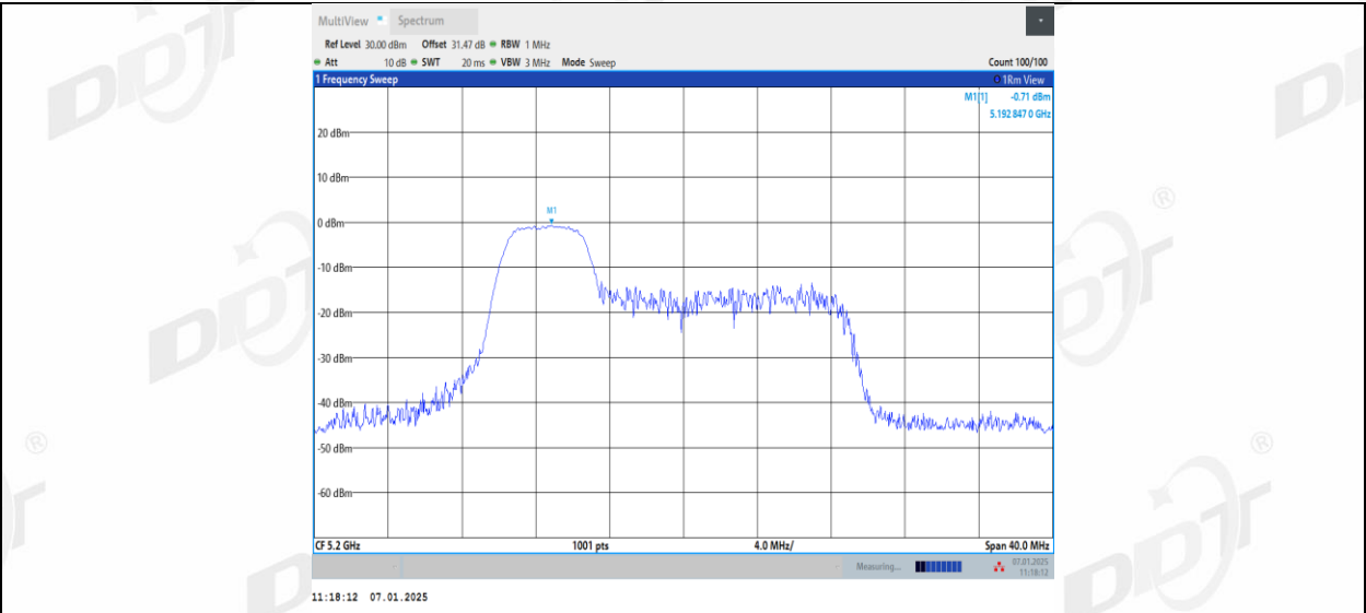
11AX20MIMO_Ant2_5200_52Tone_RU39
