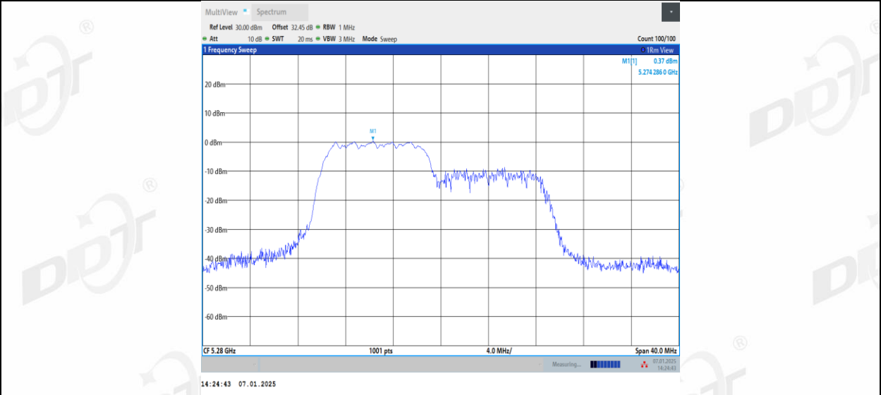
11AX20MIMO_Ant1_5280_106Tone_RU54
