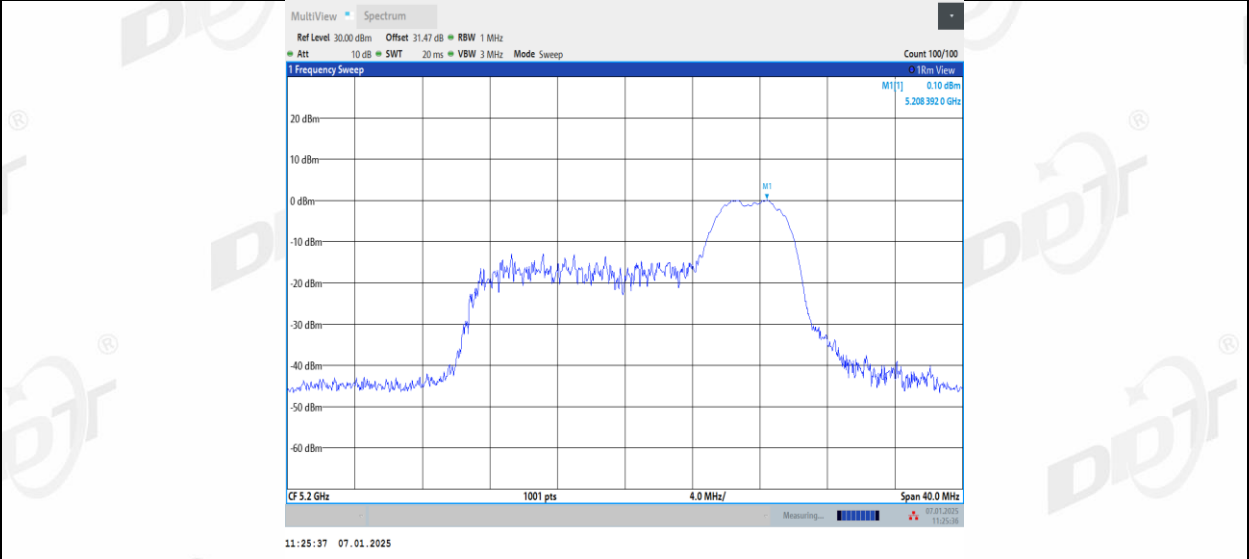
11AX20MIMO_Ant2_5200_106Tone_RU53
