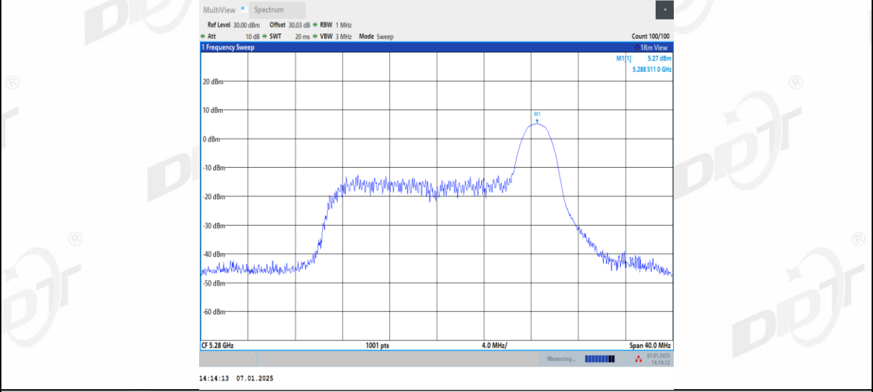
11AX20MIMO_Ant2_5280_52Tone_RU37
