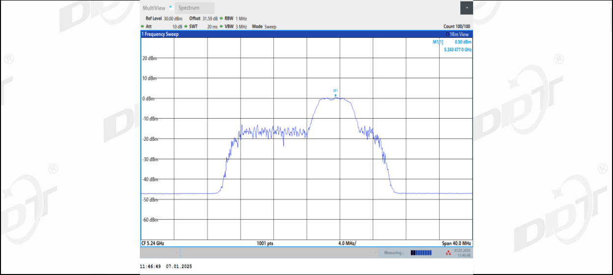
11AX20MIMO_Ant2_5240_52Tone_RU40
