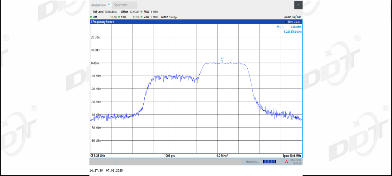
11AX20MIMO_Ant2_5280_26Tone_RU0
