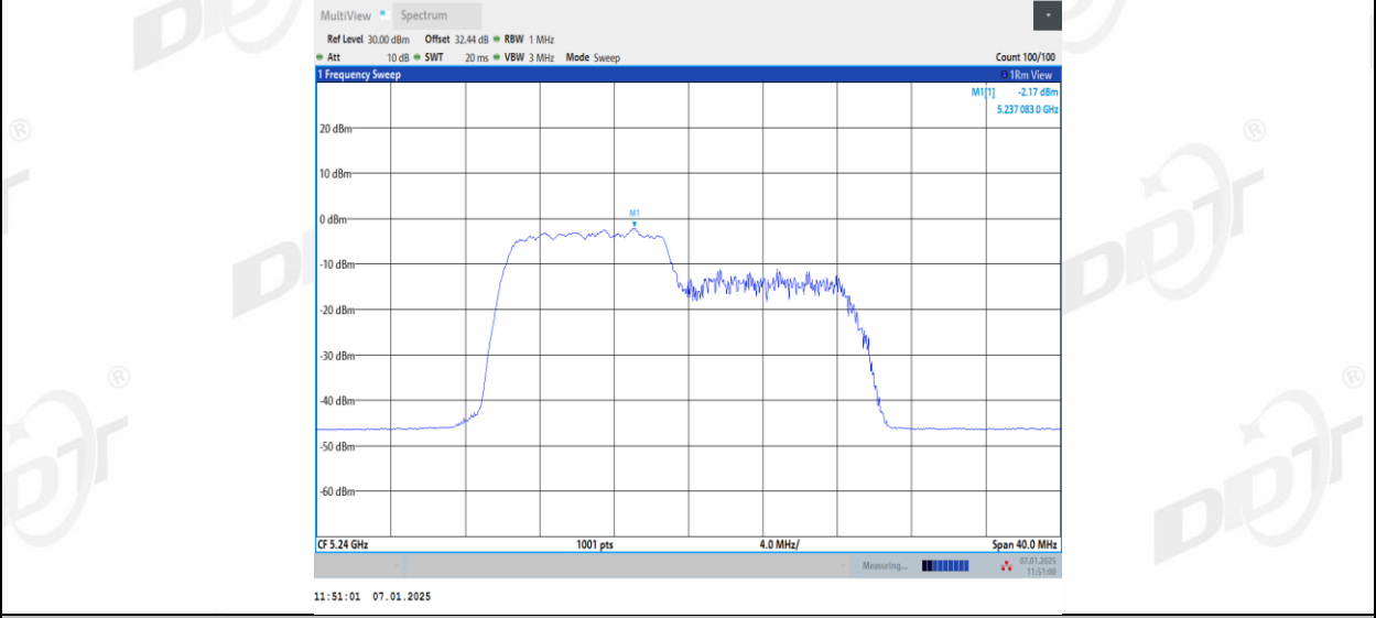
11AX20MIMO_Ant1_5240_106Tone_RU54
