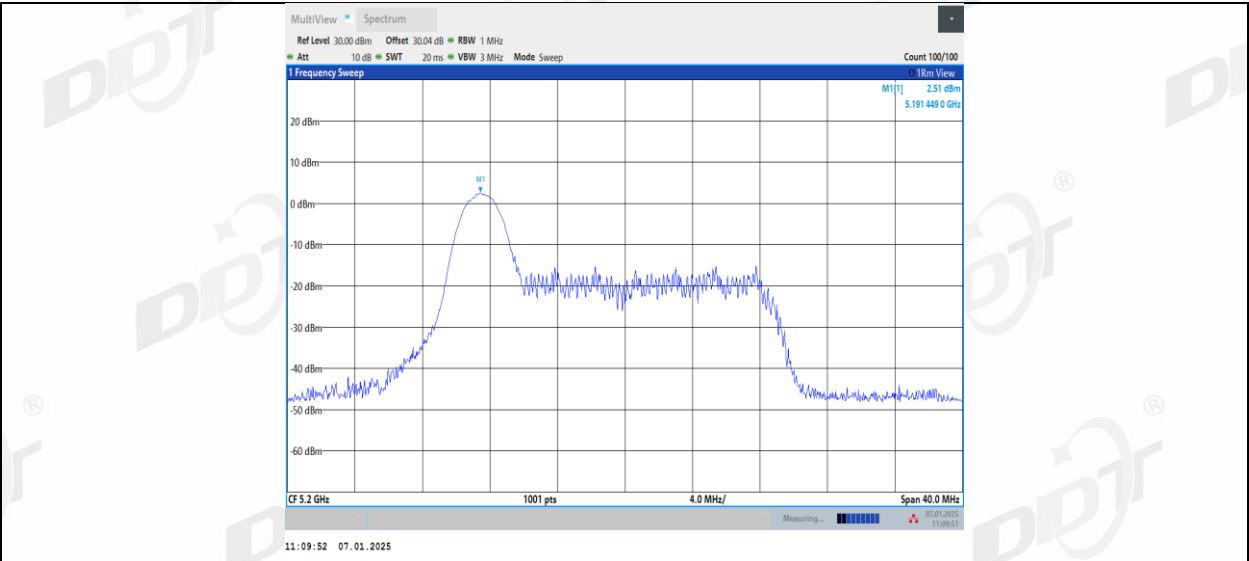
11AX20MIMO_Ant2_5200_26Tone_RU4
