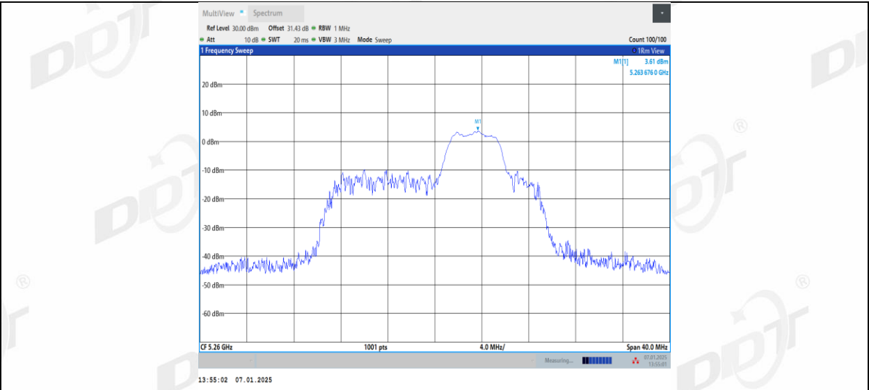
11AX20MIMO_Ant2_5260_52Tone_RU40
