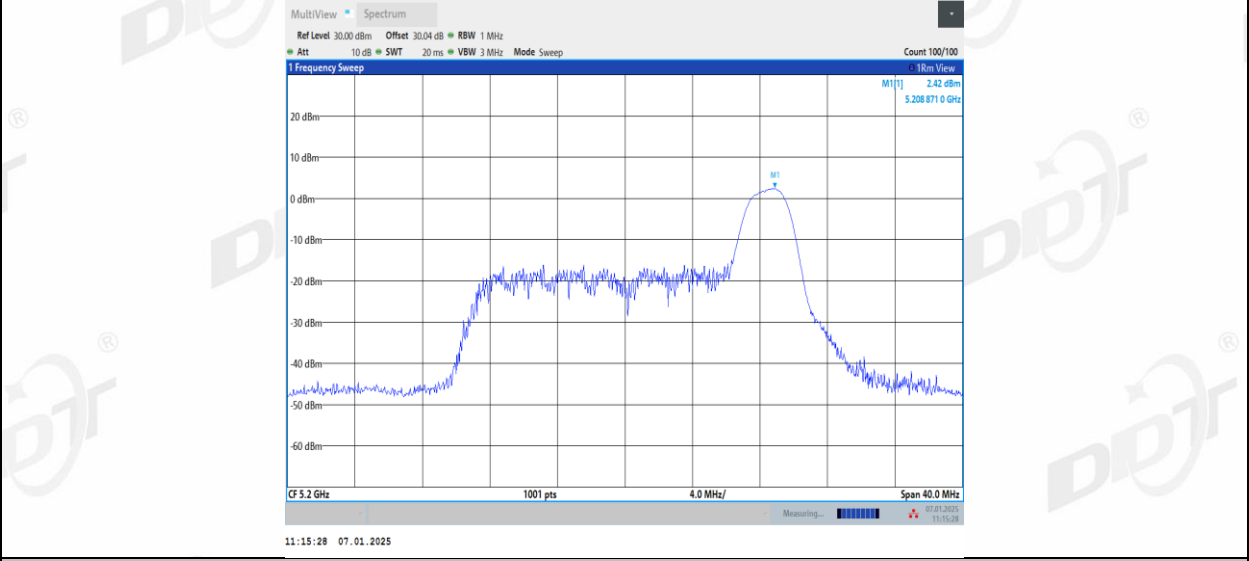
11AX20MIMO_Ant2_5200_52Tone_RU37
