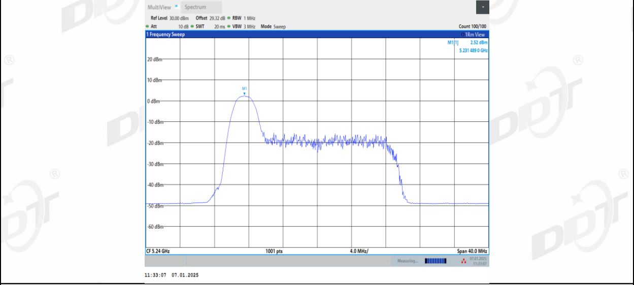
11AX20MIMO_Ant1_5240_26Tone_RU4
