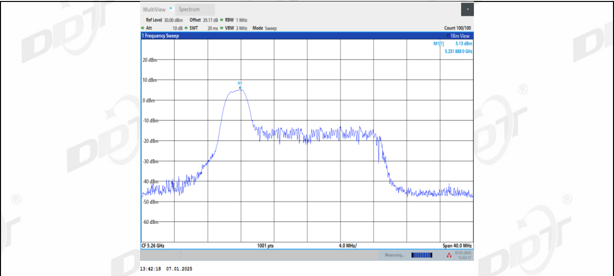
11AX20MIMO_Ant1_5260_26Tone_RU4
