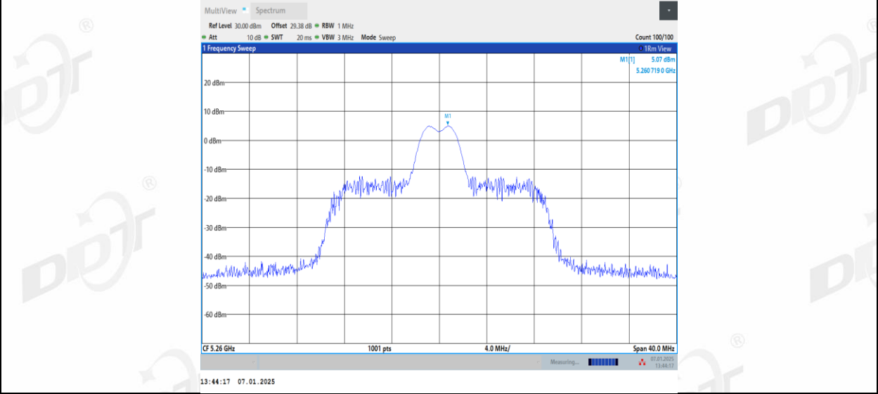
11AX20MIMO_Ant1_5260_26Tone_RU8
