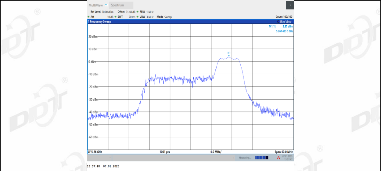
11AX20MIMO_Ant2_5260_106Tone_RU53
