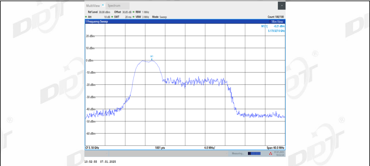
11AX20MIMO_Ant1_5180_52Tone_RU39
