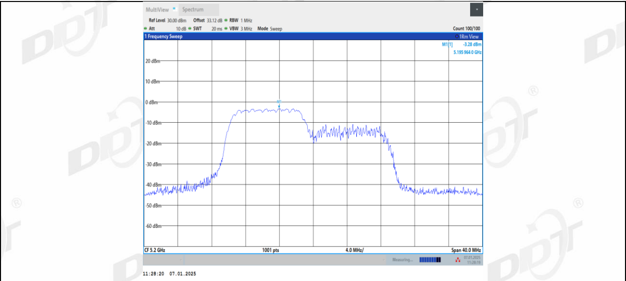
11AX20MIMO_Ant2_5200_106Tone_RU54
