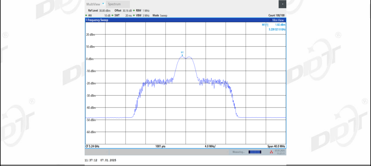
11AX20MIMO_Ant2_5240_26Tone_RU8
