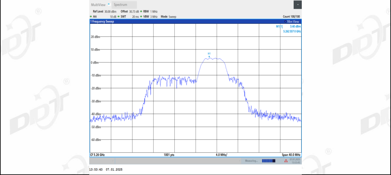
11AX20MIMO_Ant1_5260_52Tone_RU40
