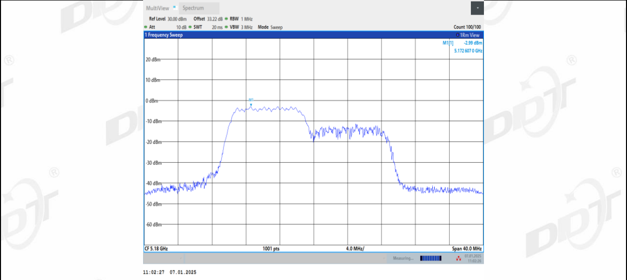
11AX20MIMO_Ant2_5180_106Tone_RU54
