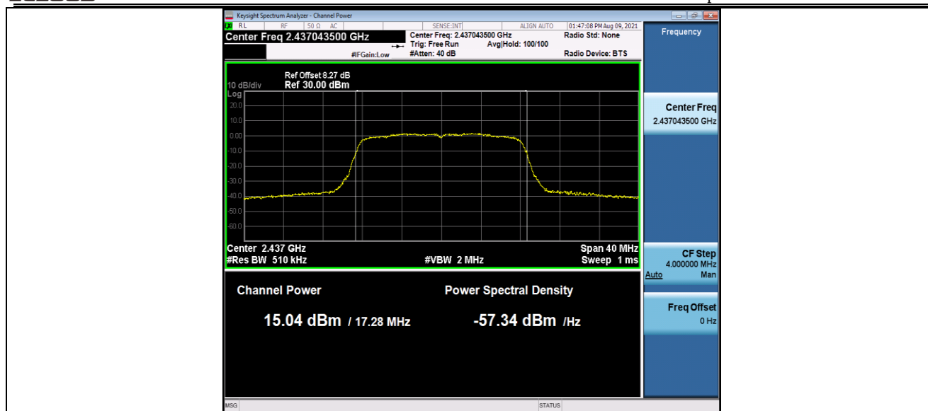
11G_Ant1_2437
