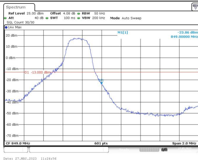
Band5-3MHz-QPSK-20635-15RB#0
