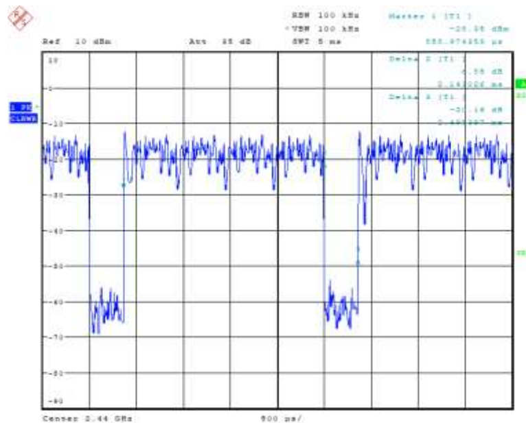
Fig.26. Duty cycle: BLE 2440 MHz
