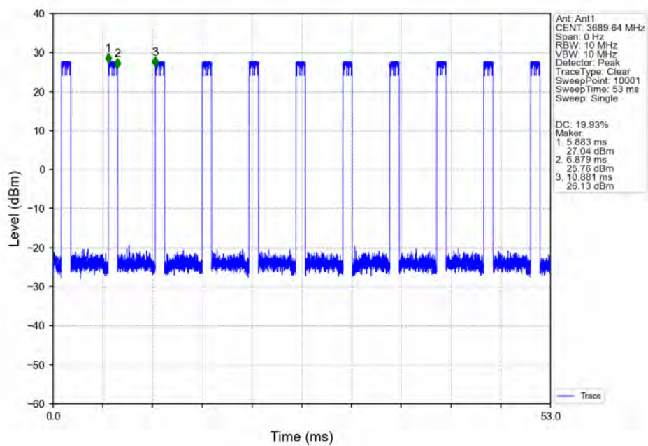
n48_30kHz_SISO_NTNV_20MHz_DFT-s-OFDM_16_QAM_3690MHz_Inner_Full_Ant1
