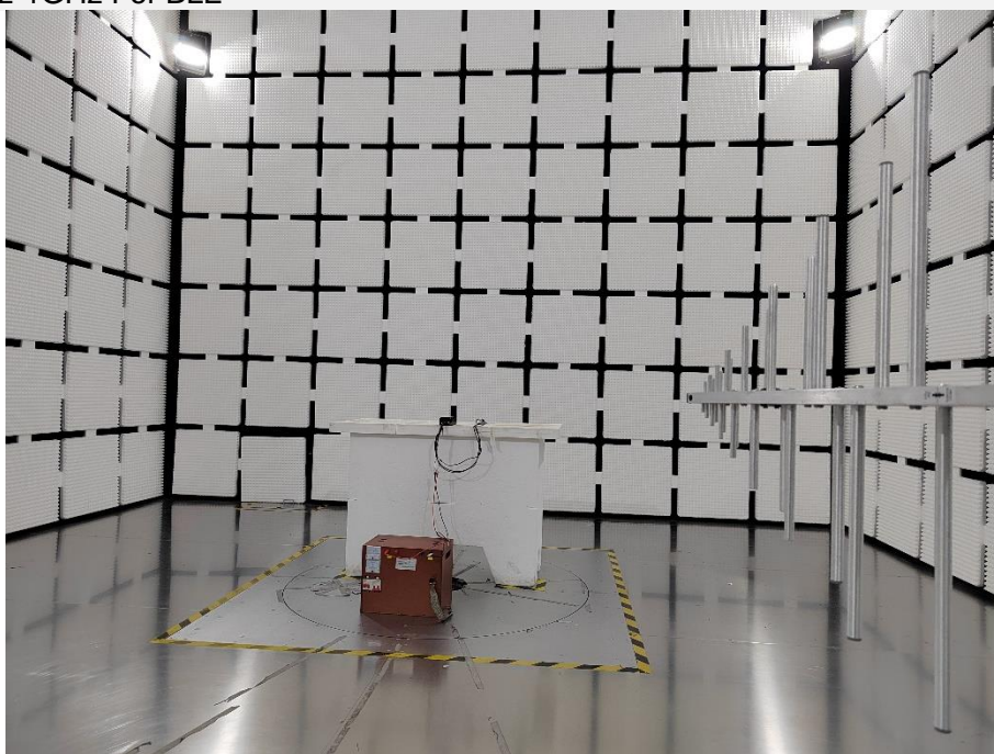
30MHz-1GHz For BLE
