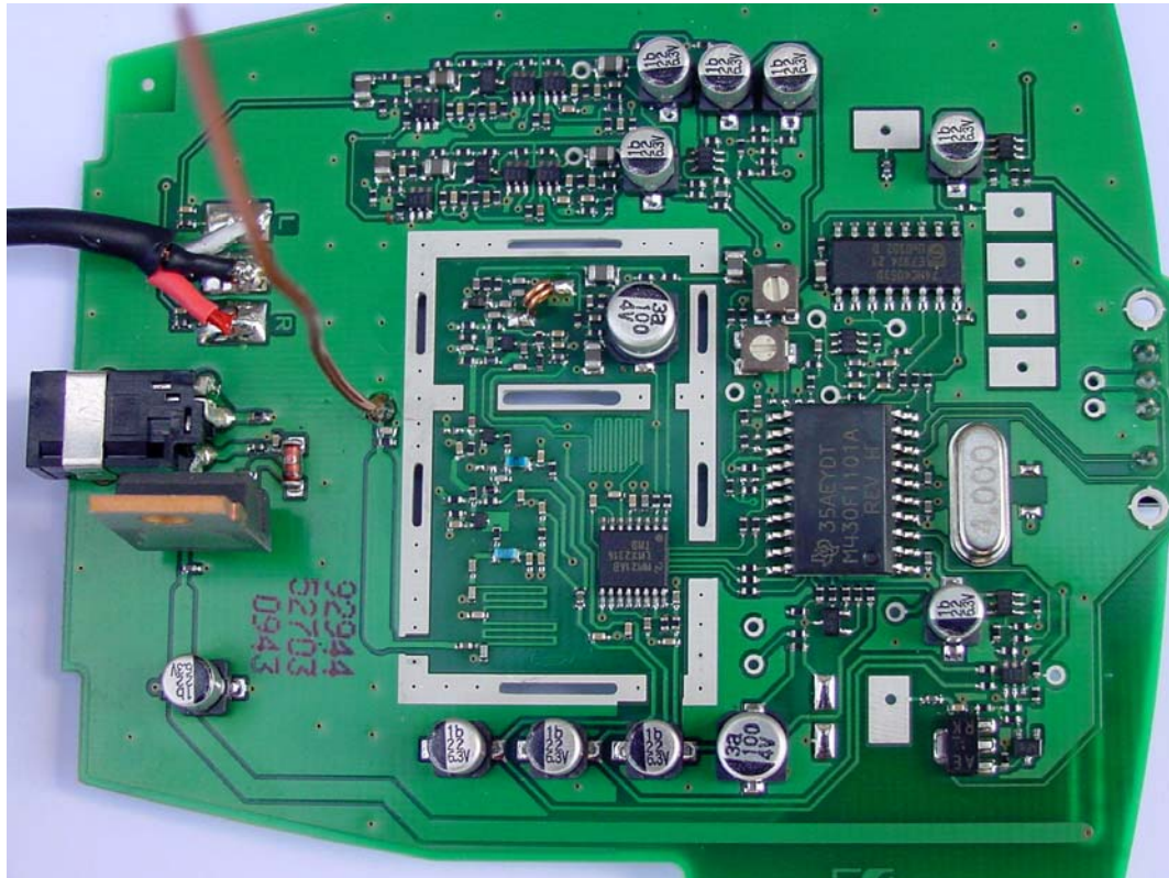
PCB TR110/120
