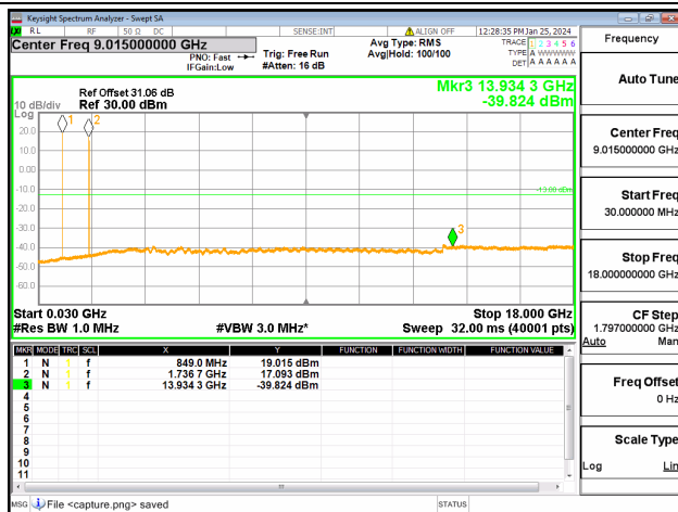
4A-5A / 20+10MHz / QPSK / High+High CH / 1@0-1@49
